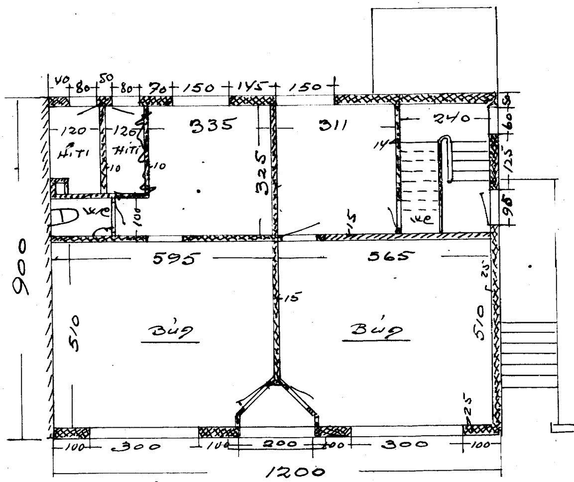
1. HÆÐ
