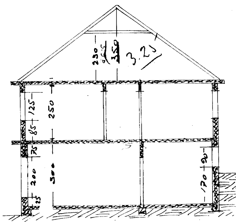
SKURÐUR
