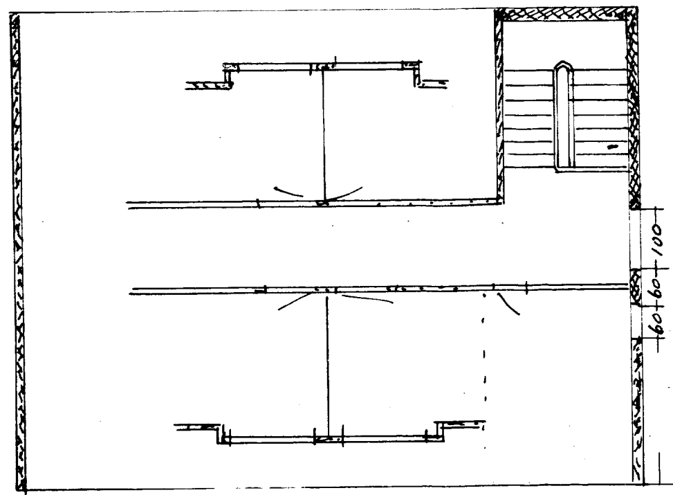
FORHAFIÐ
