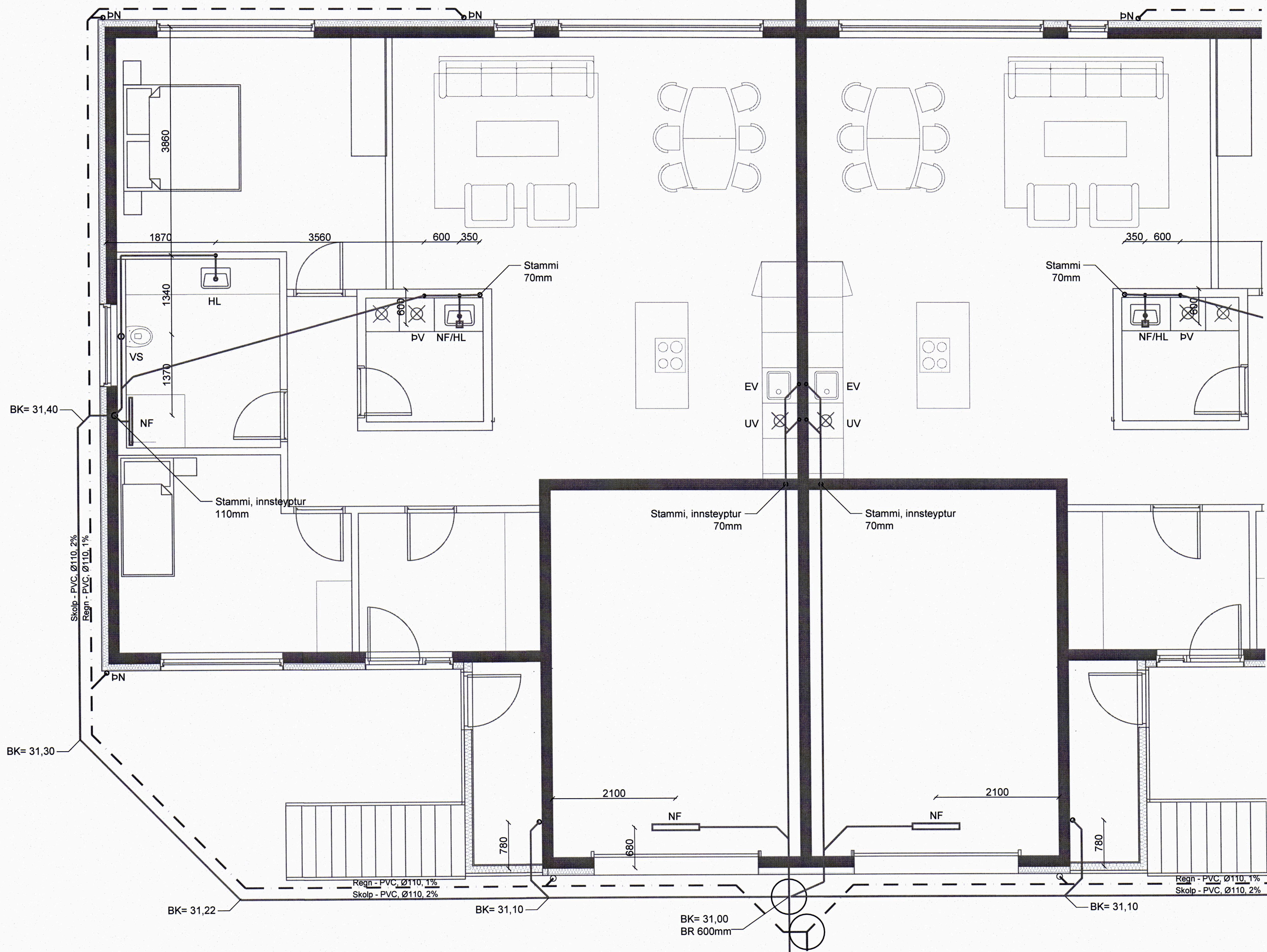
Grunnmynd frárennslis, 1. hæð 1:50
