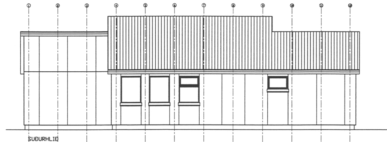
ÞUDURHLIÐ
