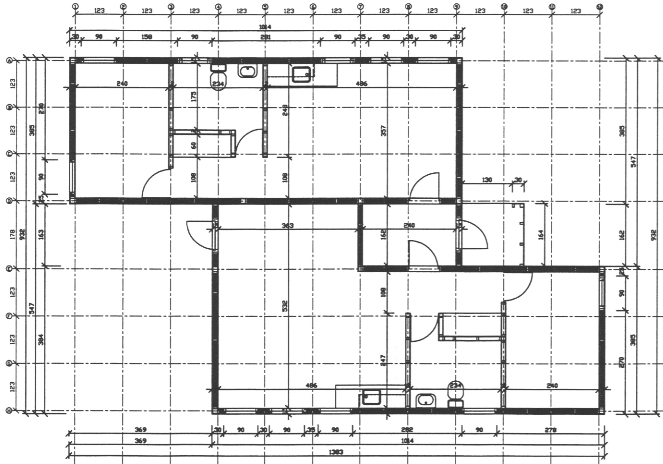
GRUNNMYND
