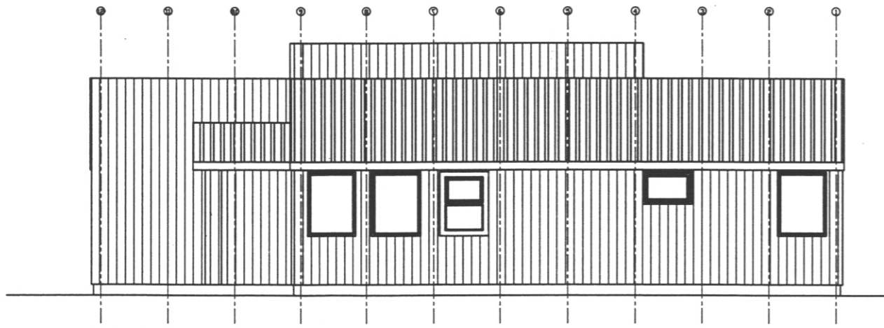
NORÐURHLIÐ
