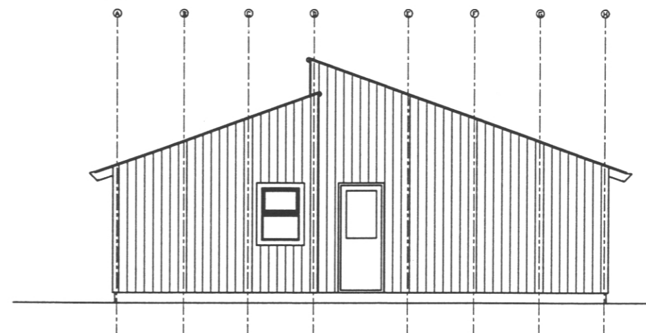
VESTURHLIÐ
