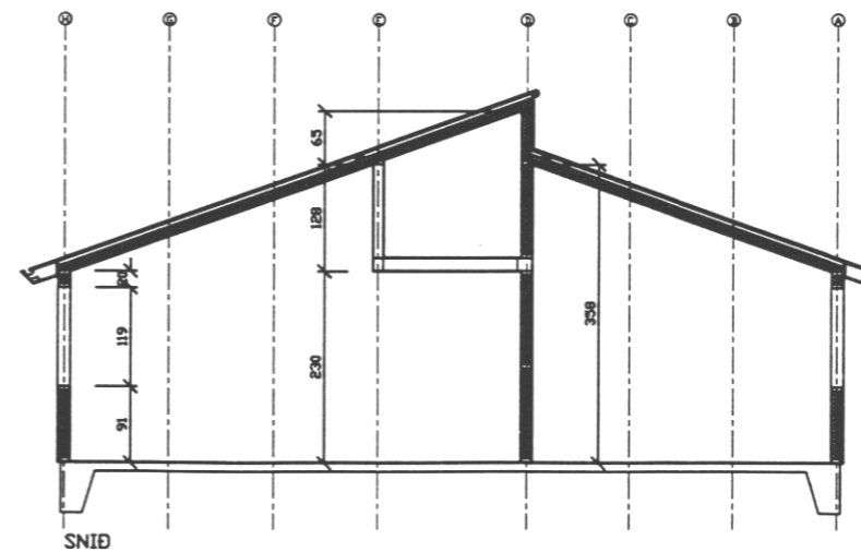
SNIÐ
