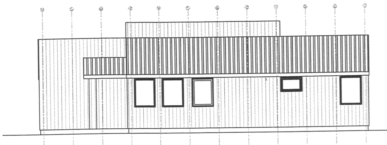
NORÐURHLID
