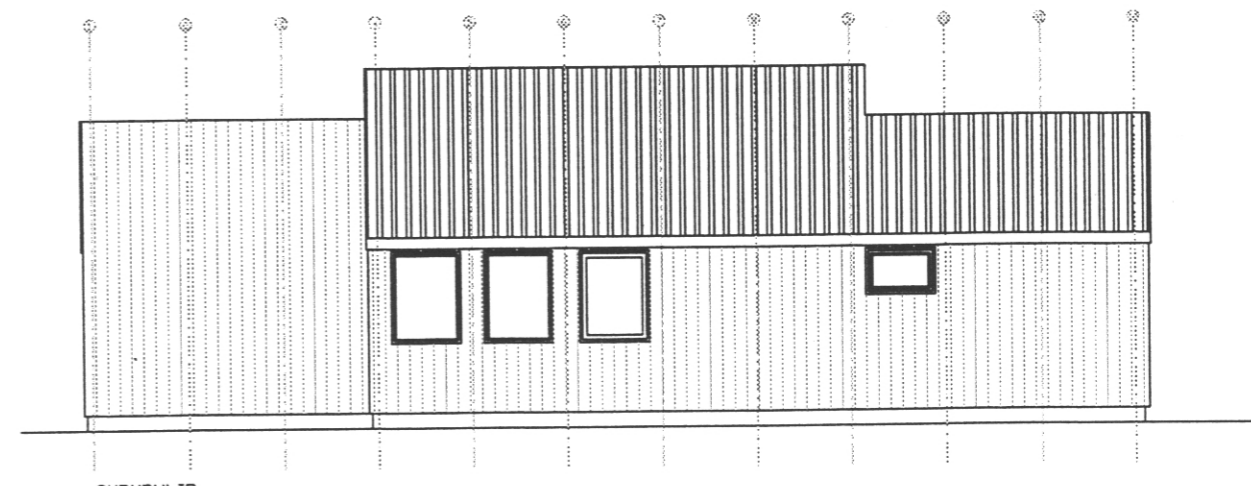
SUDURHLID
