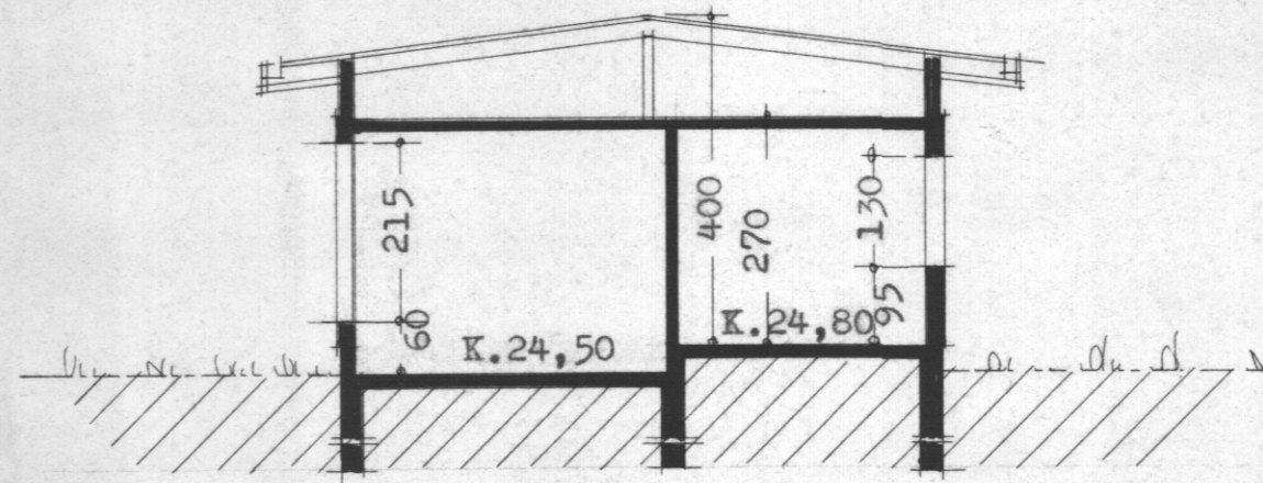
skurður A-A
