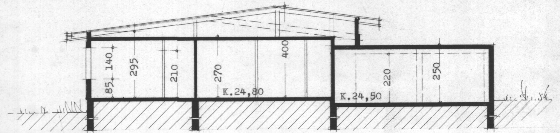
skurður B-B
