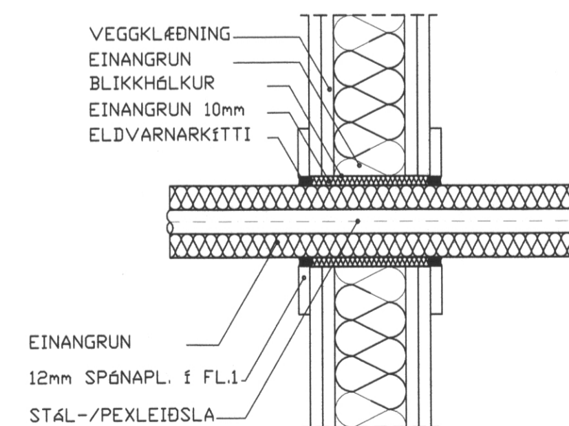
FRÁGANGUR Á STÁL-/PEXLEIÐSLU GEGNUM LÉTTAN VEGG
