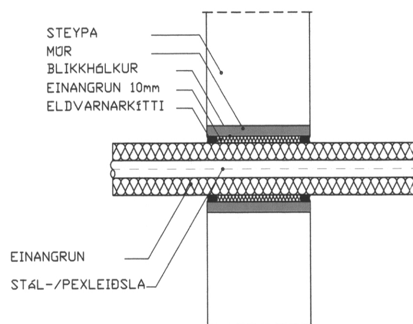
FRÁGANGUR Á STÁL-/PEXLEIÐSLU GEGNUM STEYPTAN VEGG
