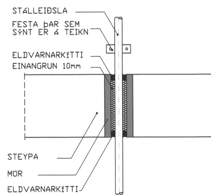
FRÁGANGUR Á STÁLLEIÐSLU GEGNUM STEYPT GÓLF
