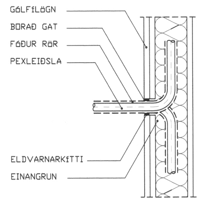
BRUNABÉTTING Á PEXLEIÐSLU Í FÓÐURRÖRI Í GEGNUM KLÆÐNINGU
