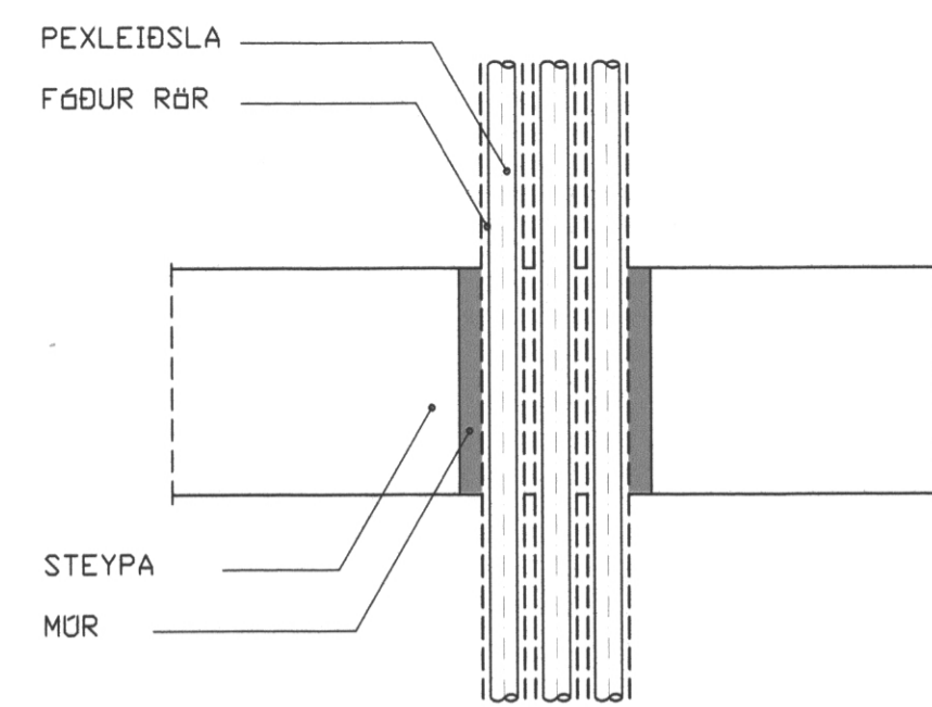
FRÁGANGUR Á PEXLEIÐSLU GEGNUM STEYPT GÓLF
