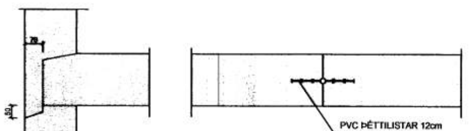
LÓÐRÉTT SNIÐ
