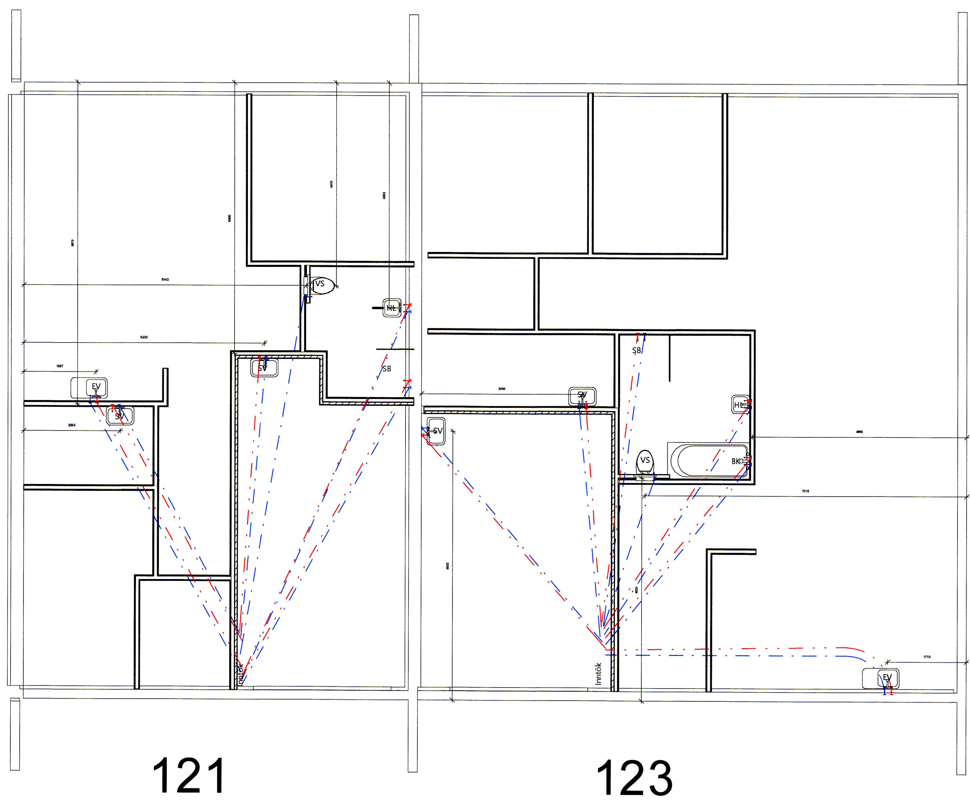
1 Grunnmynd Neysluvatn 121-123 1:50
