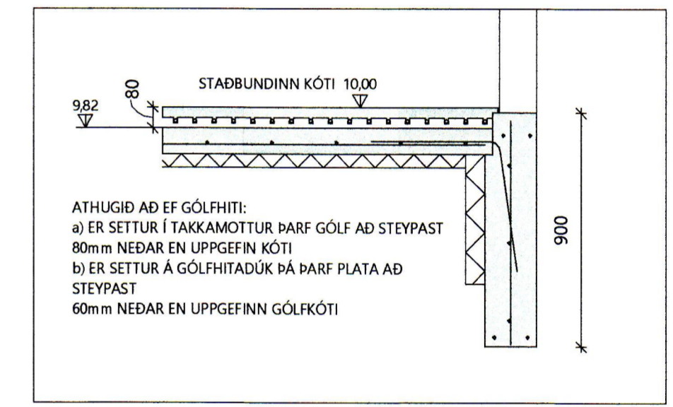
ATH Gólfhiti 1:20
