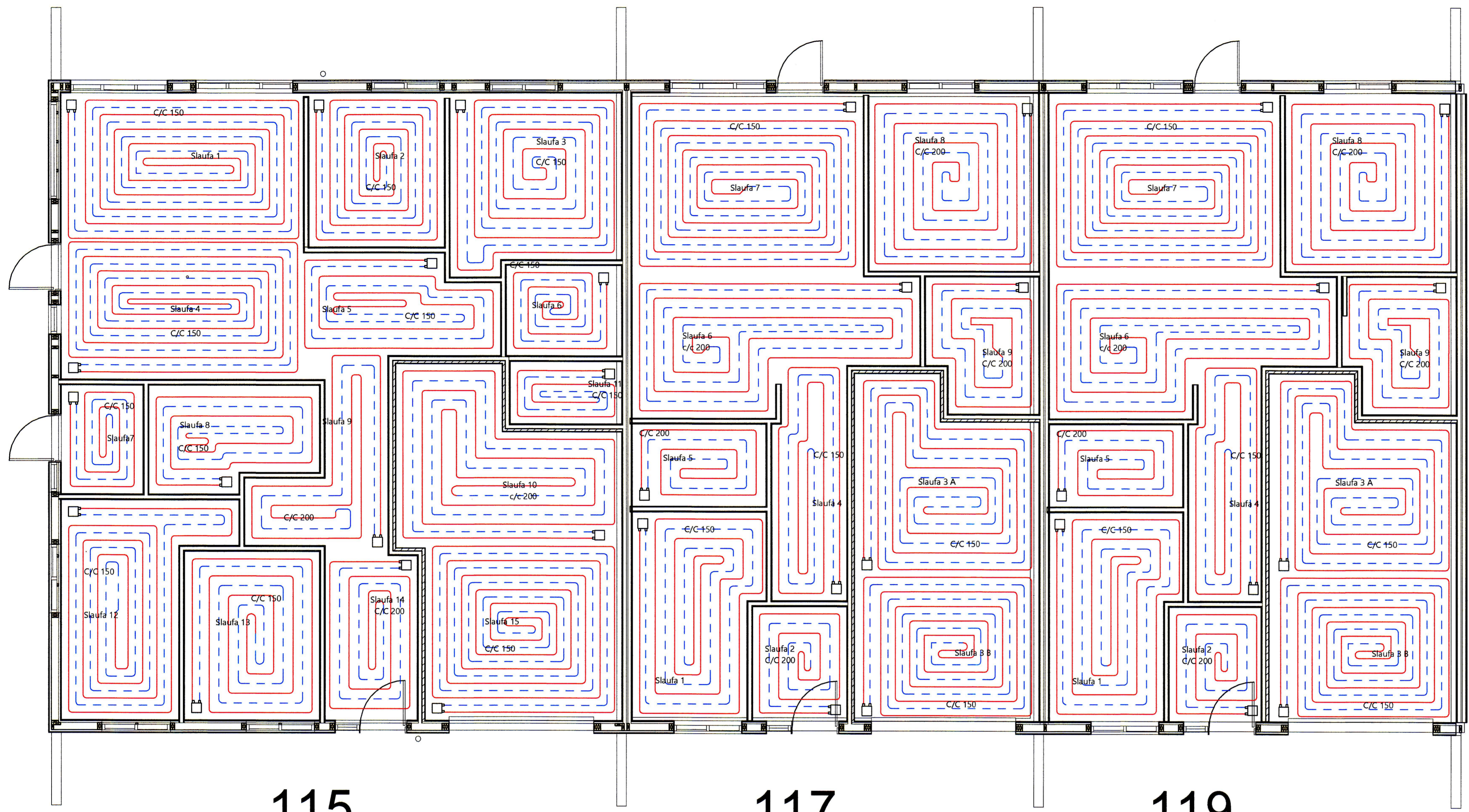
1 Grunnmynd íbúð 1 Gólfhitalagnir 115-119 1:50
