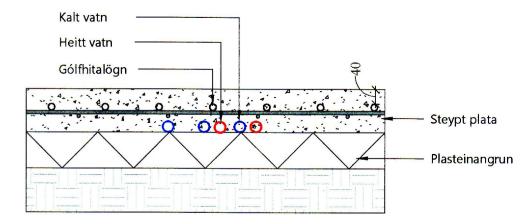
Hitalagnir í plötu 1:10
