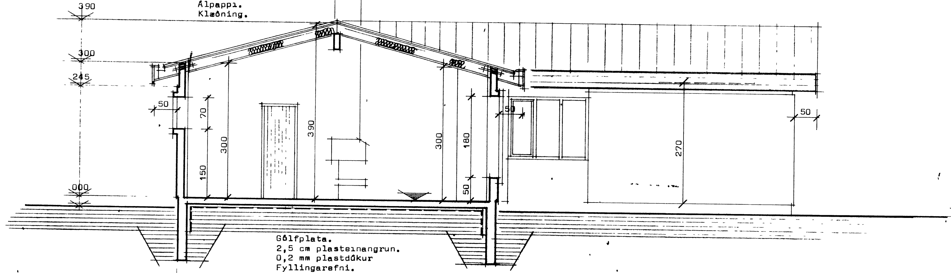
Sneiðing ... BB
