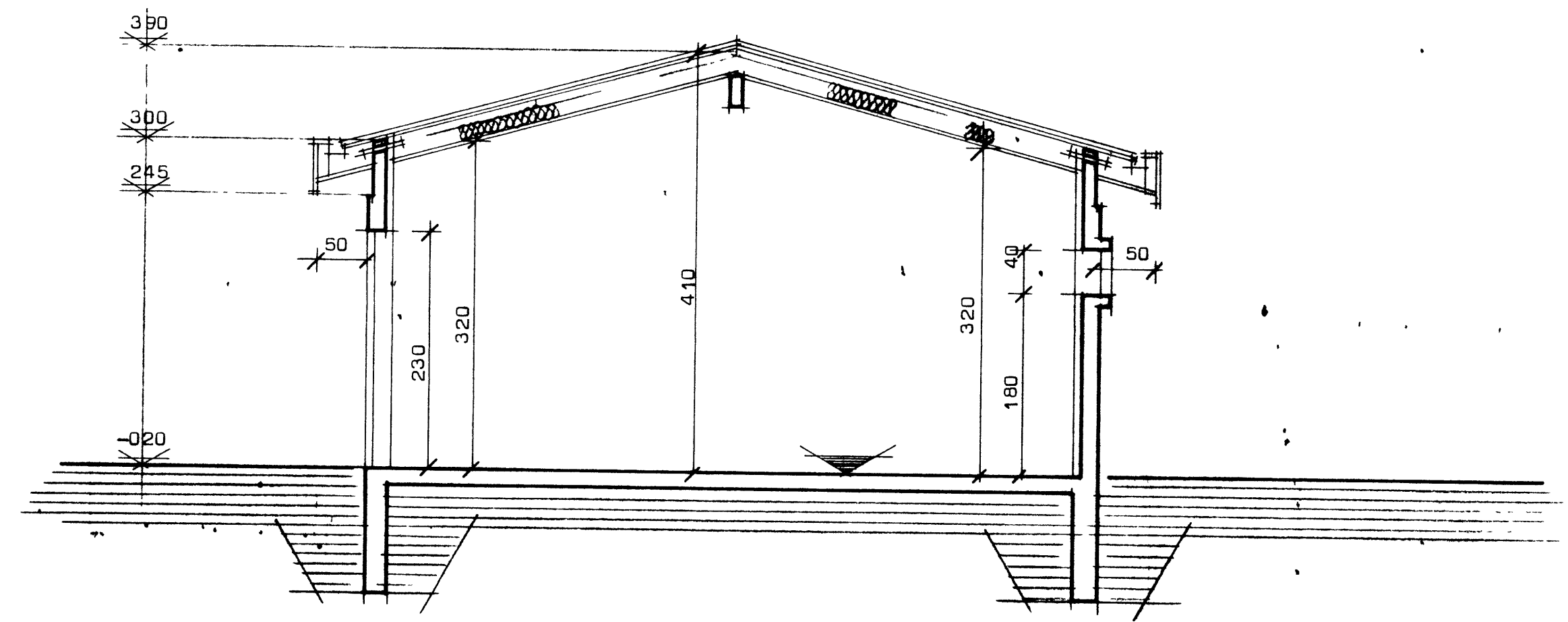
Sneiðing .... AA
