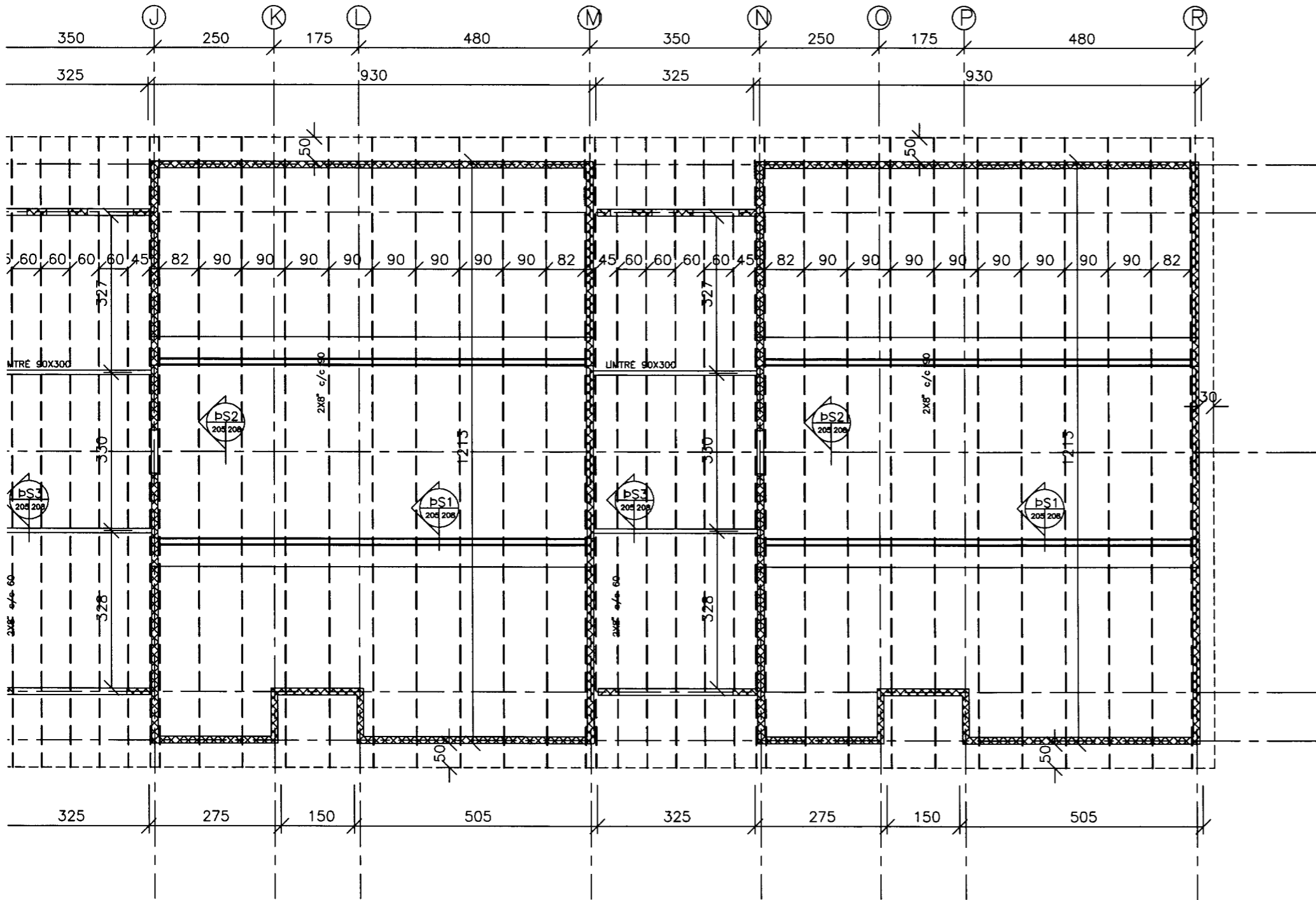
GRUNNMYND M=1:50
