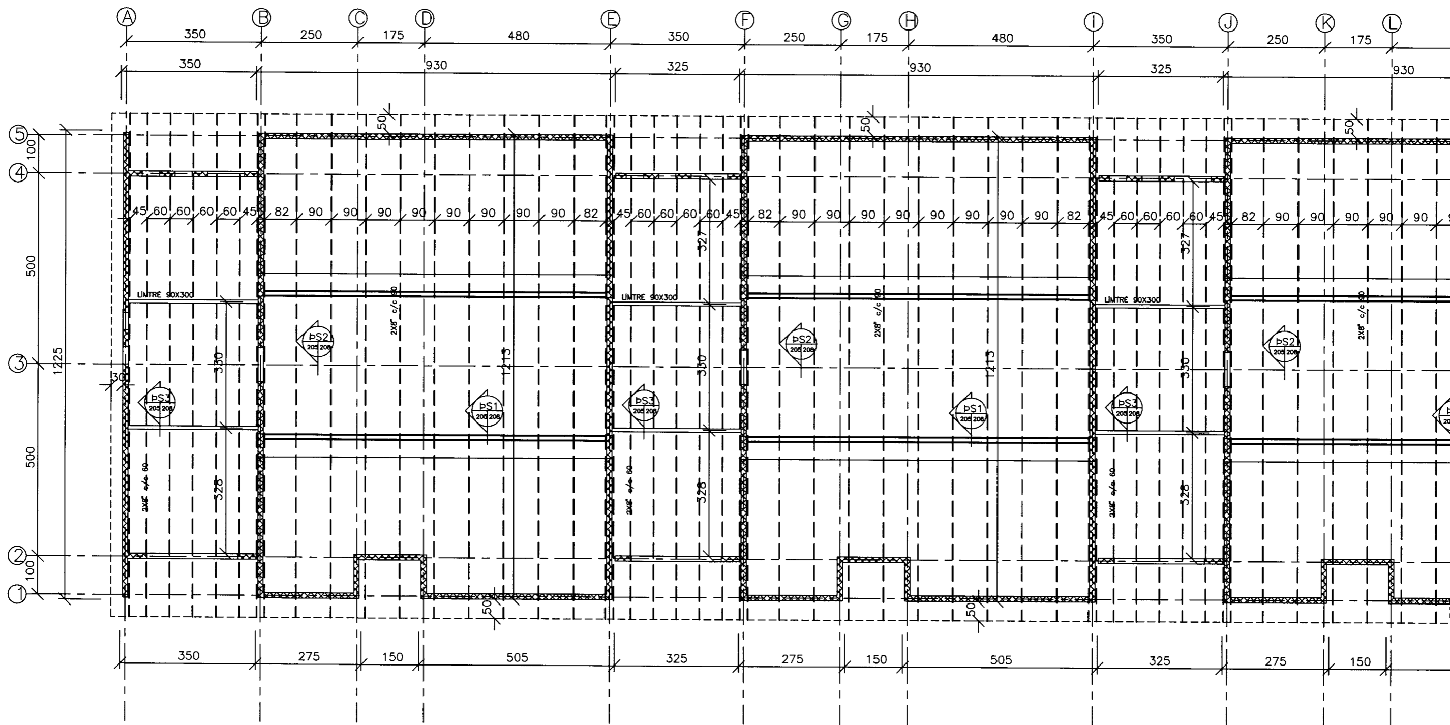
GRUNNMYND M=1:50
