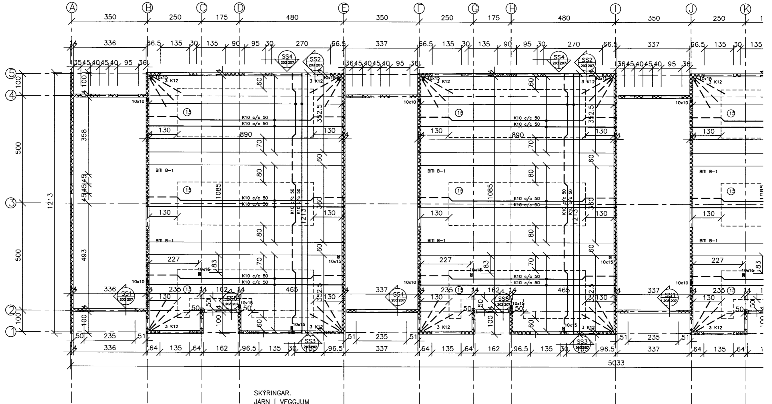
GRUNNMYND M=1:50
