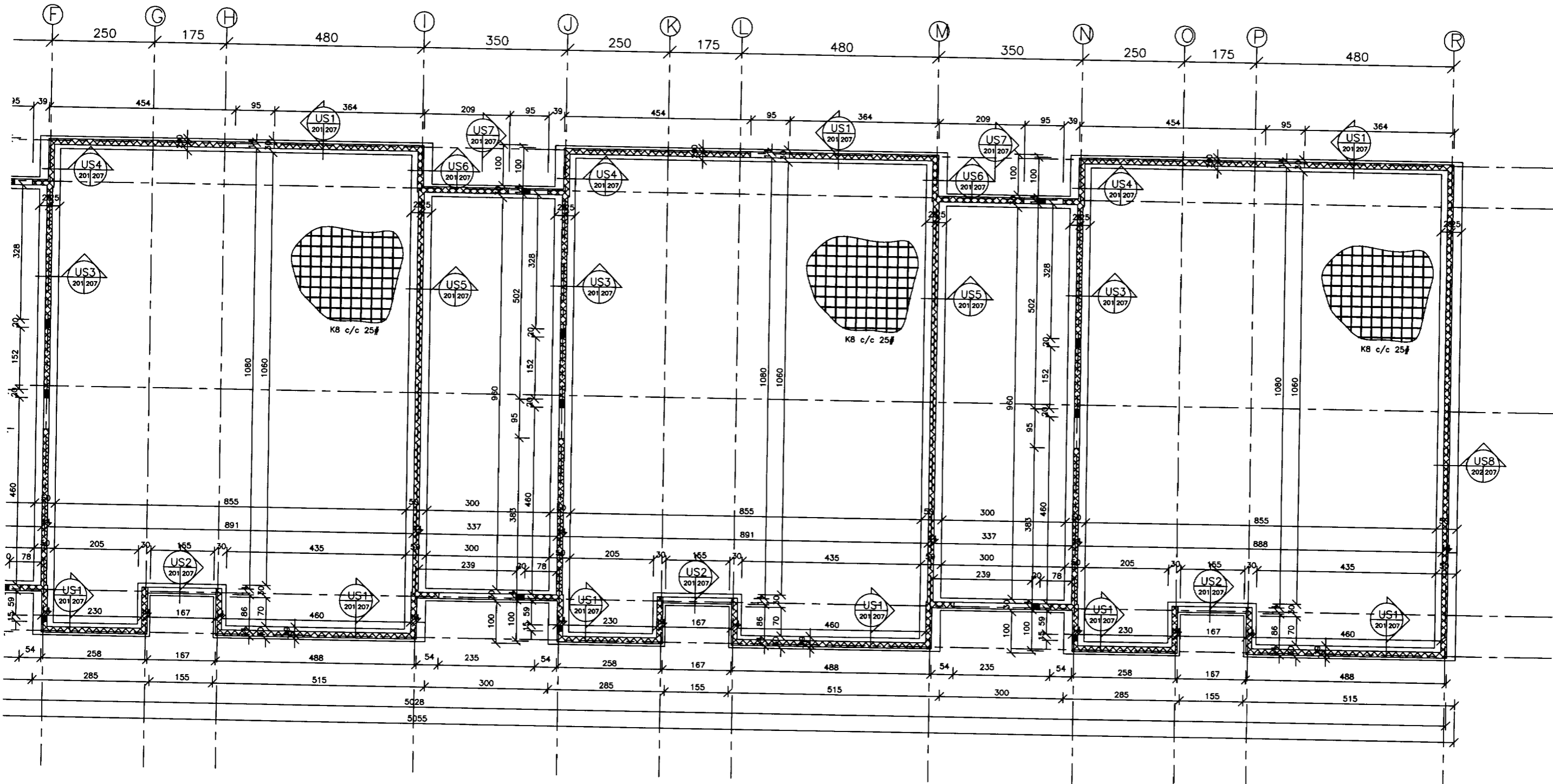
GRUNNMYND M=1:50
