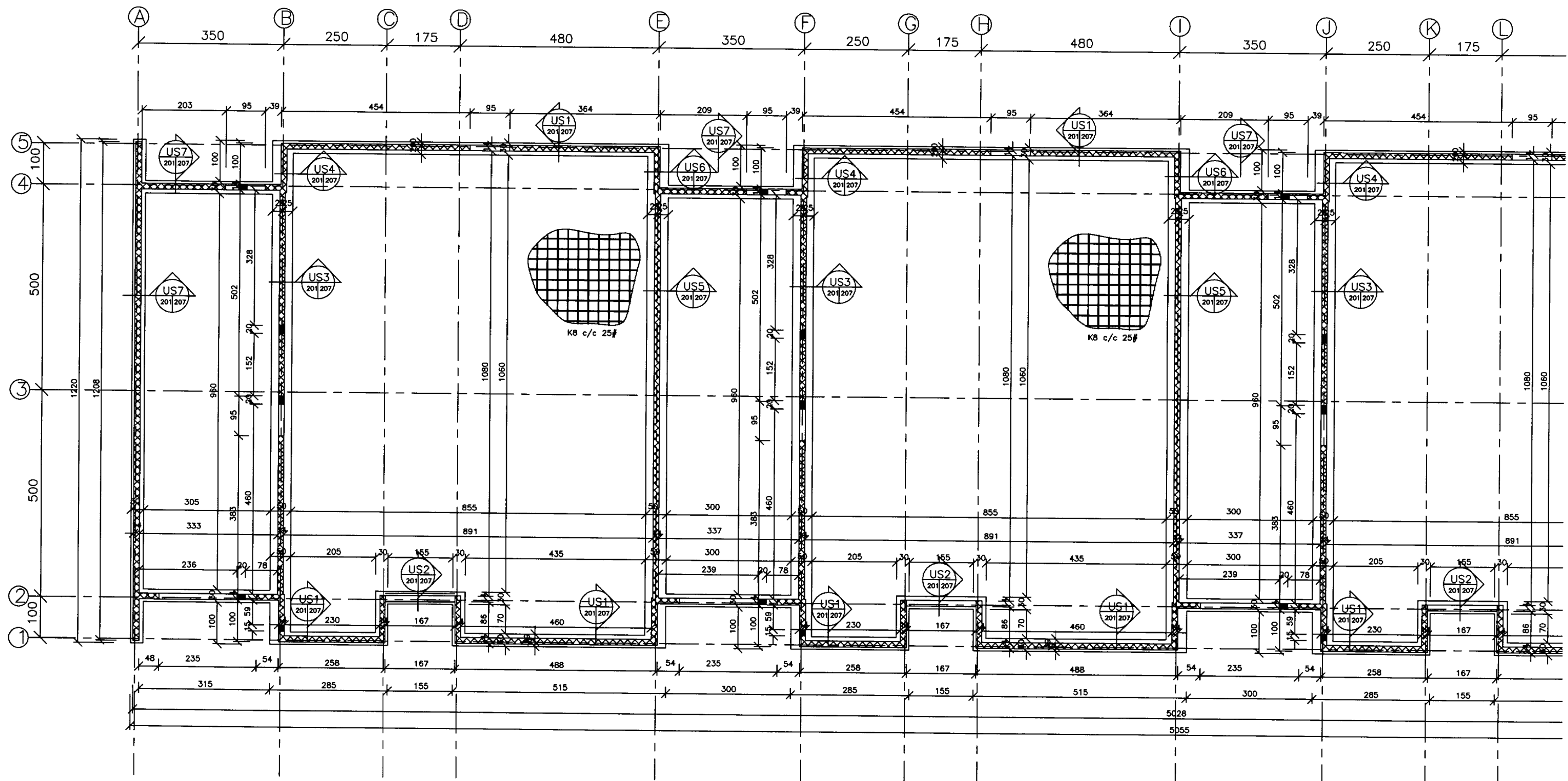
GRUNNMYND M=1:50
