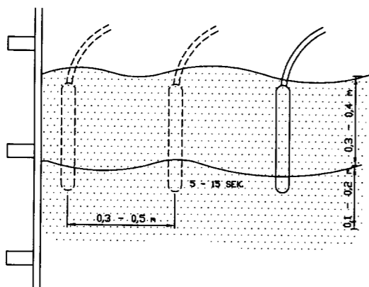
SKÝRINGAMYND: TITRAN STEYPU Í VEGG
