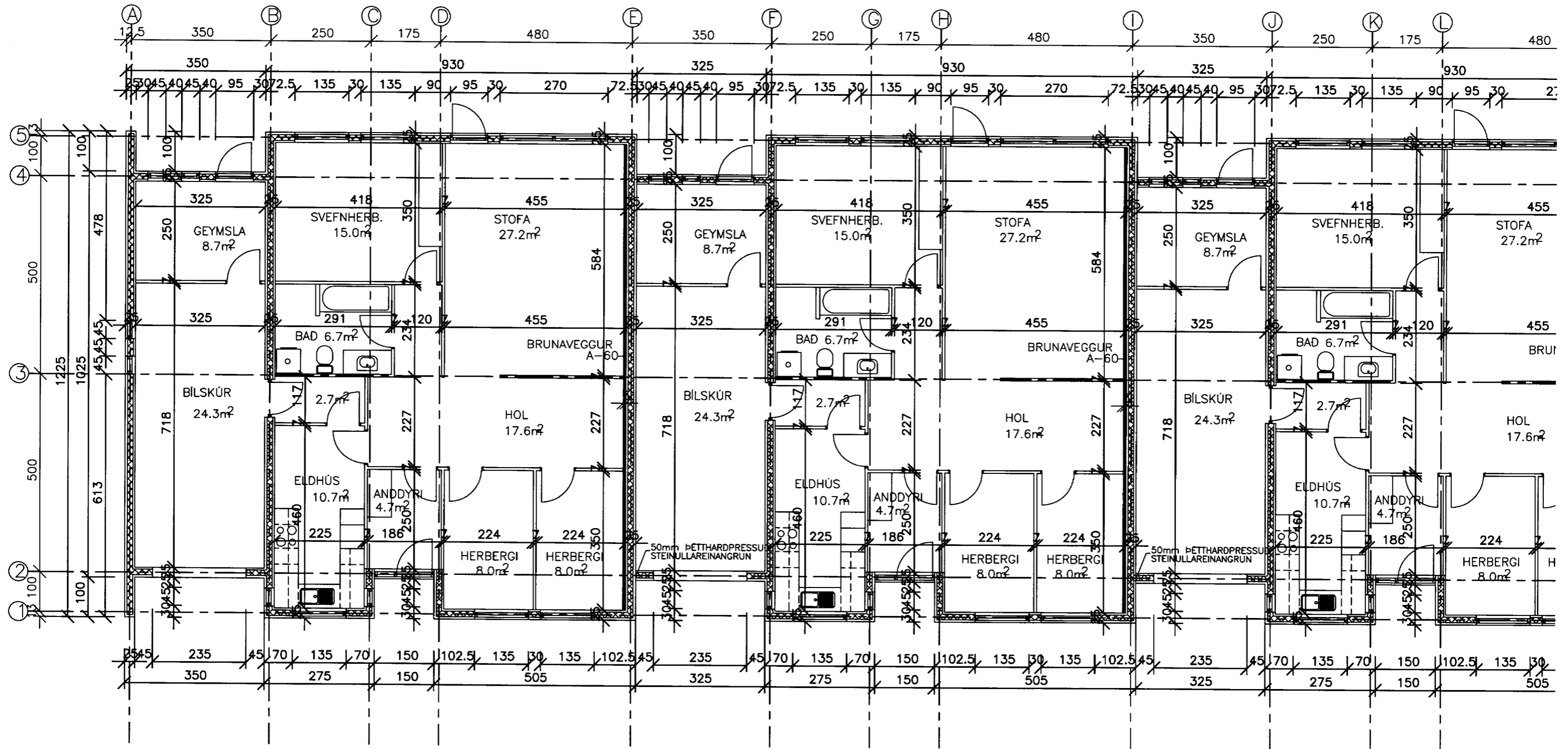
GRUNNMYND M=1:50
