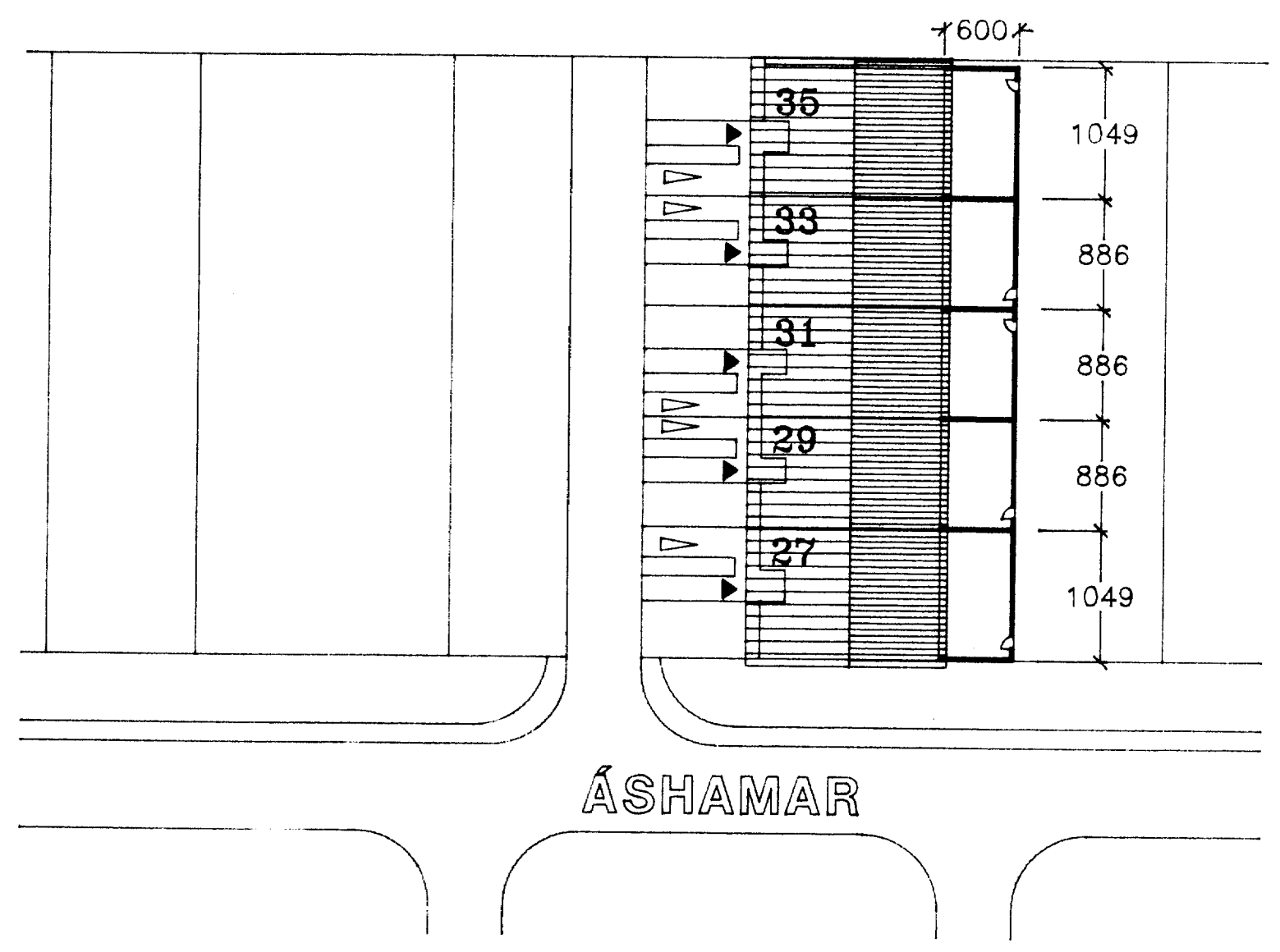
AFSTÖÐUMYND
