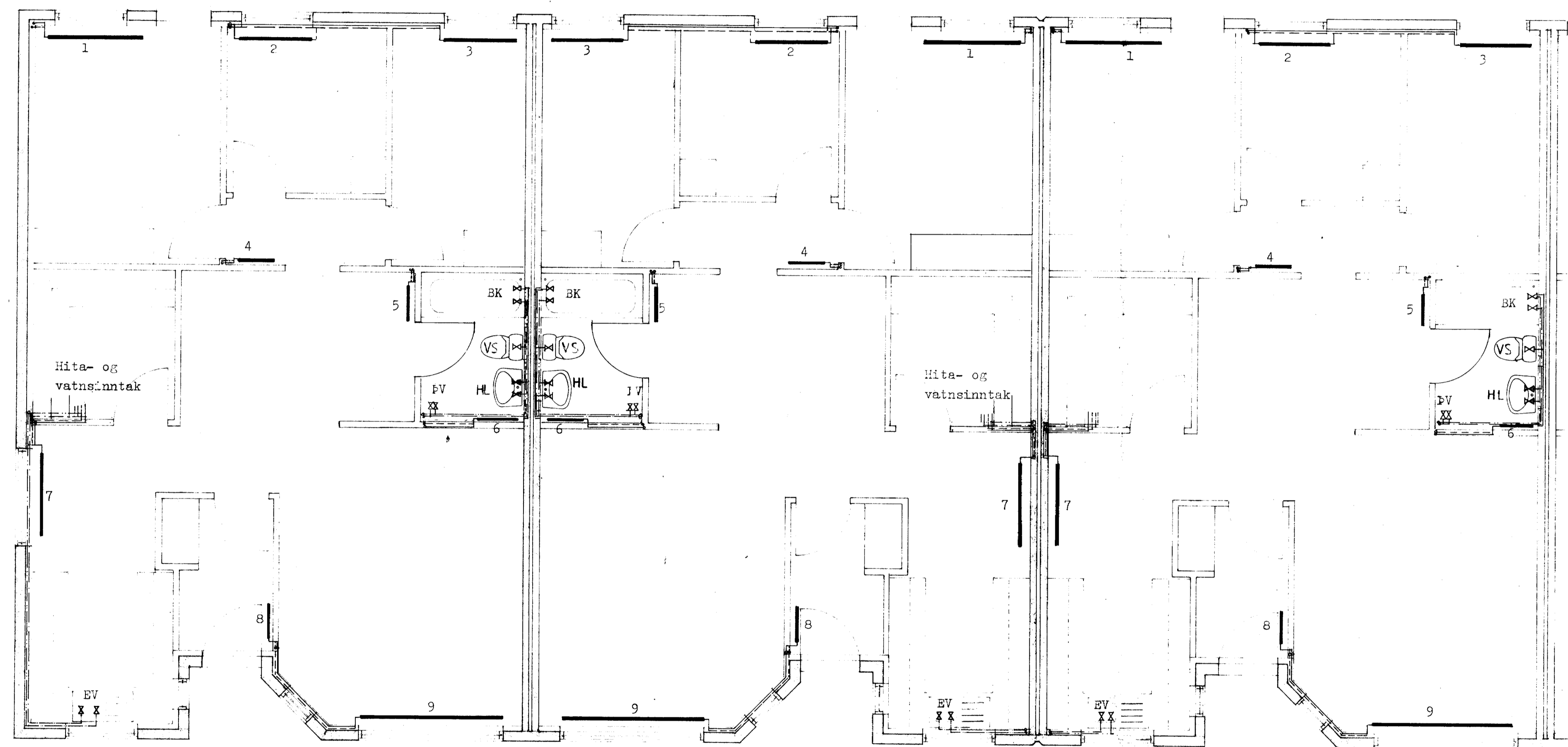
GRUNNMYND Mkv 1:50
