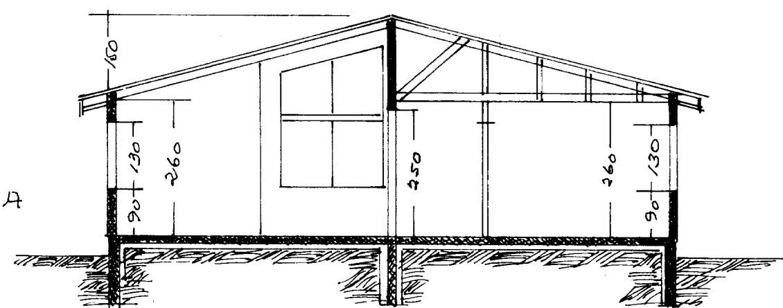
SKURÐUR A-A
