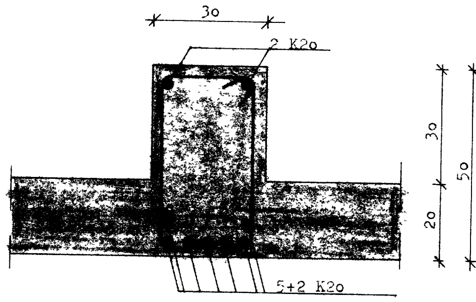
SNID A-A Mkv. 1:10
