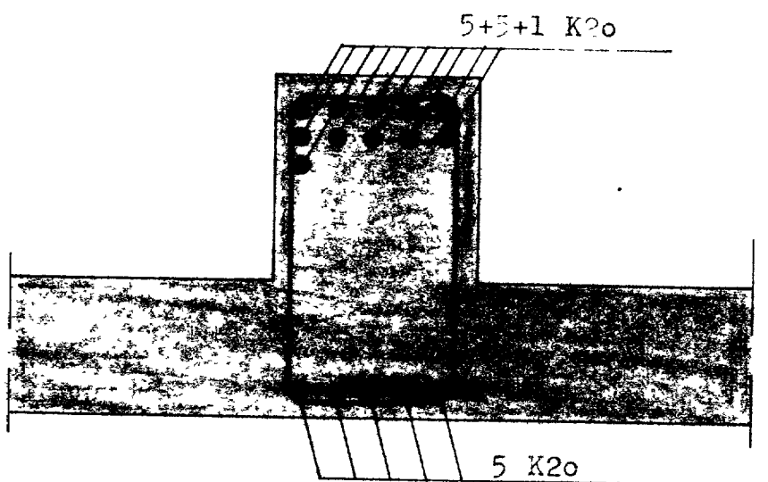
SNID B-B Mkv. 1:10
