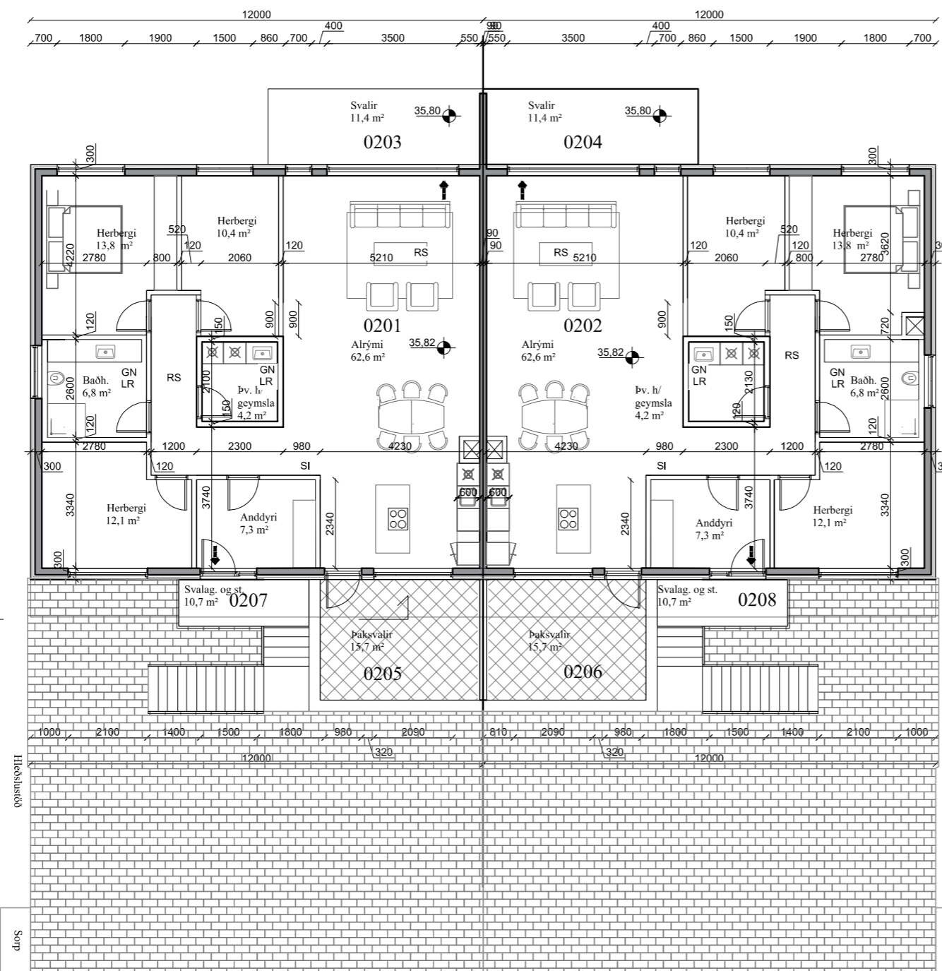
Grunnmynd 2. hæð 1:100
