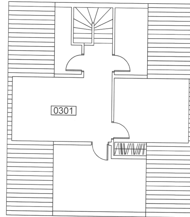
grunnmynd 3. hæð, sýnir 180cm salarhæð mkv 1:100
