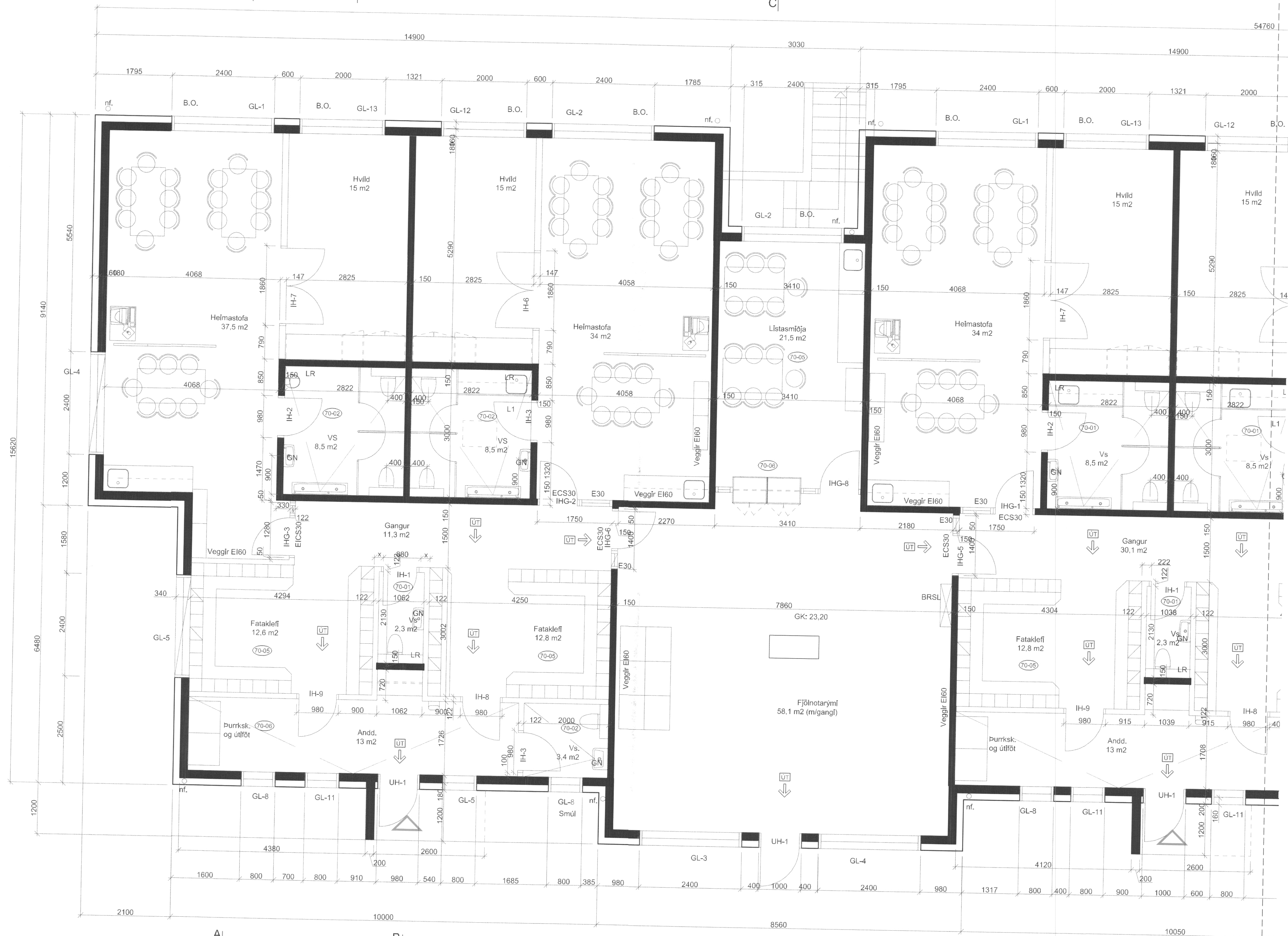
GRUNNMYND KJALLARI m.kv. 1:50
