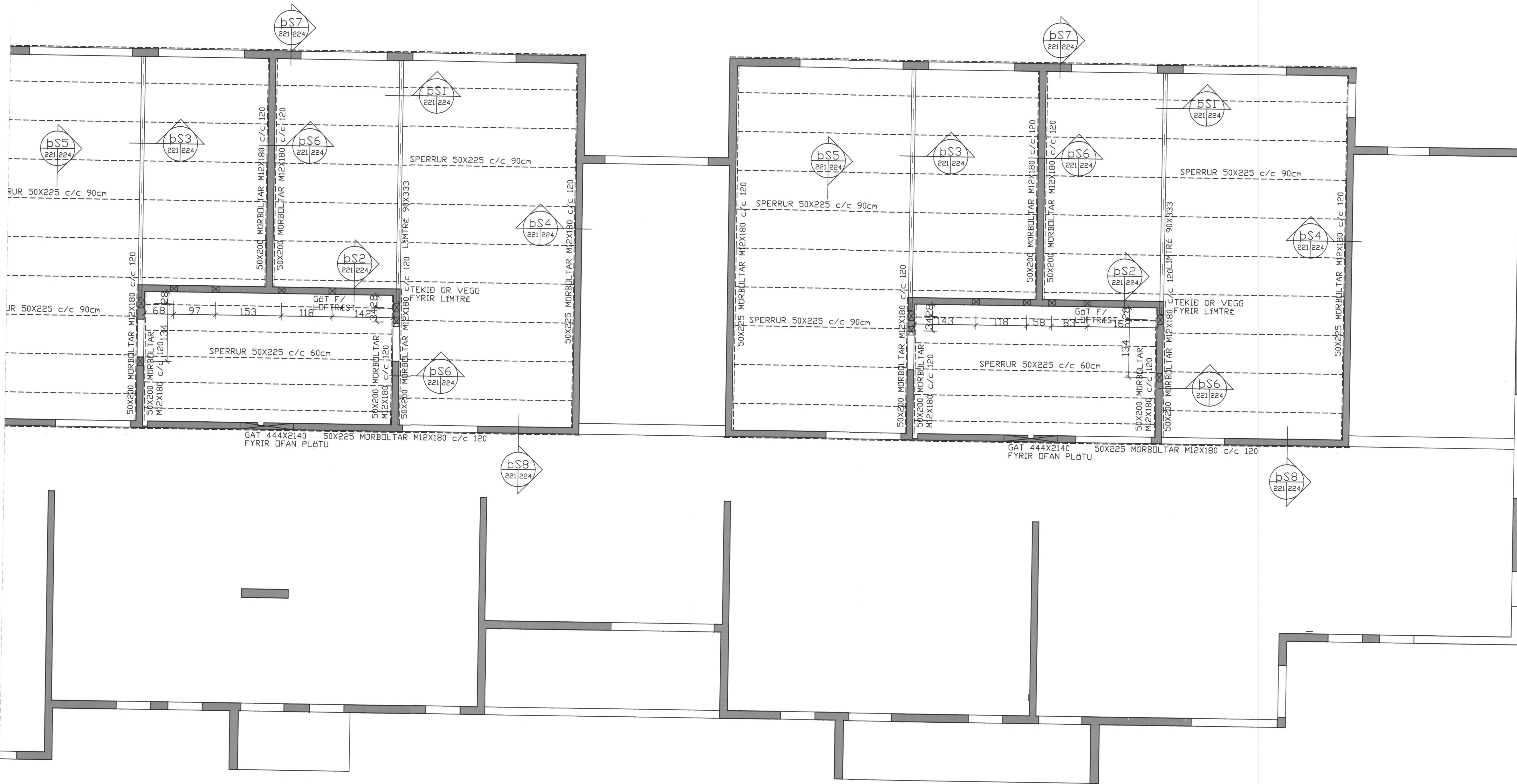
GRUNNMYND SPERRUR M=1:50
