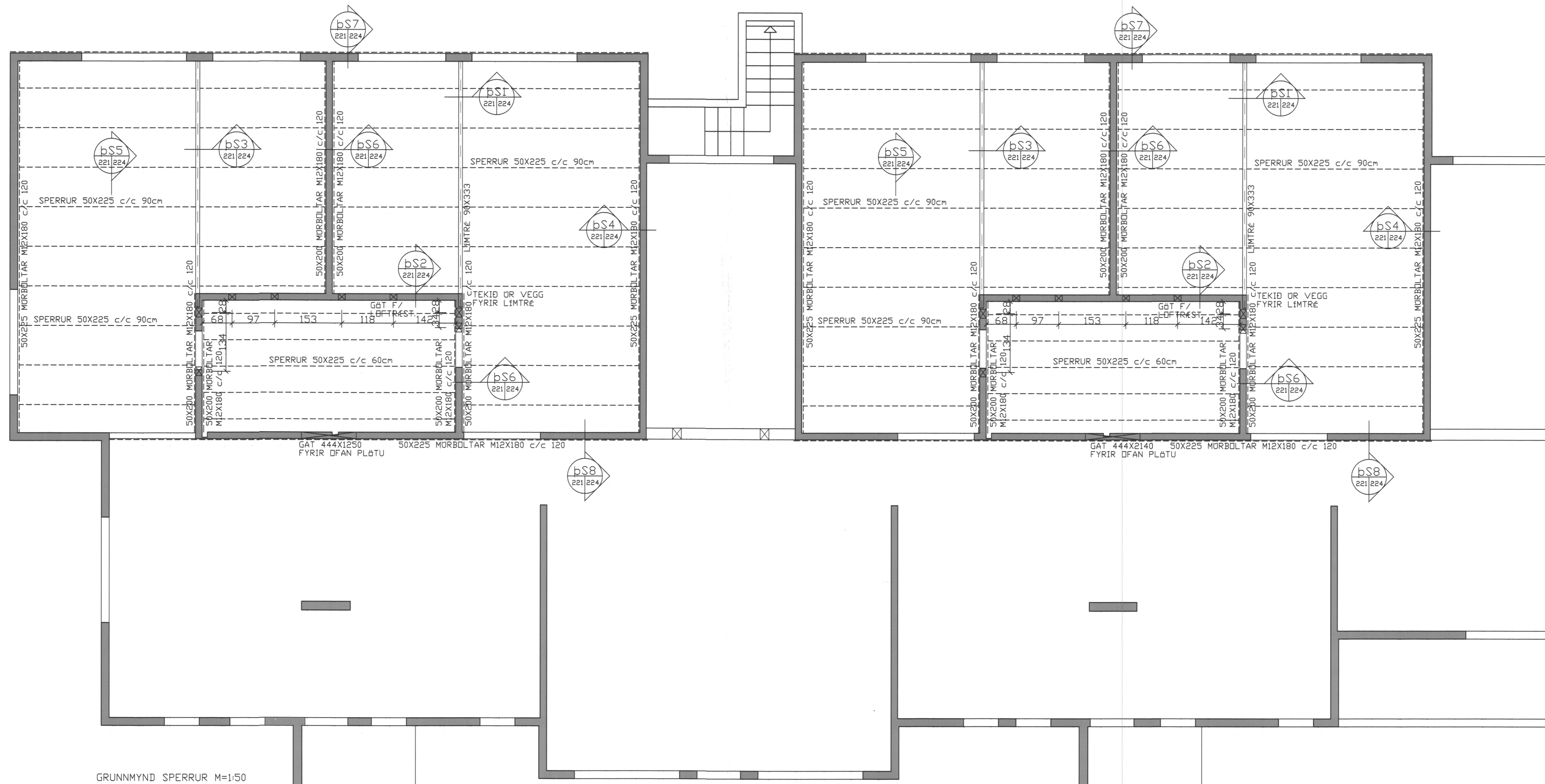
GRUNNMYND SPERRUR M=1:50
