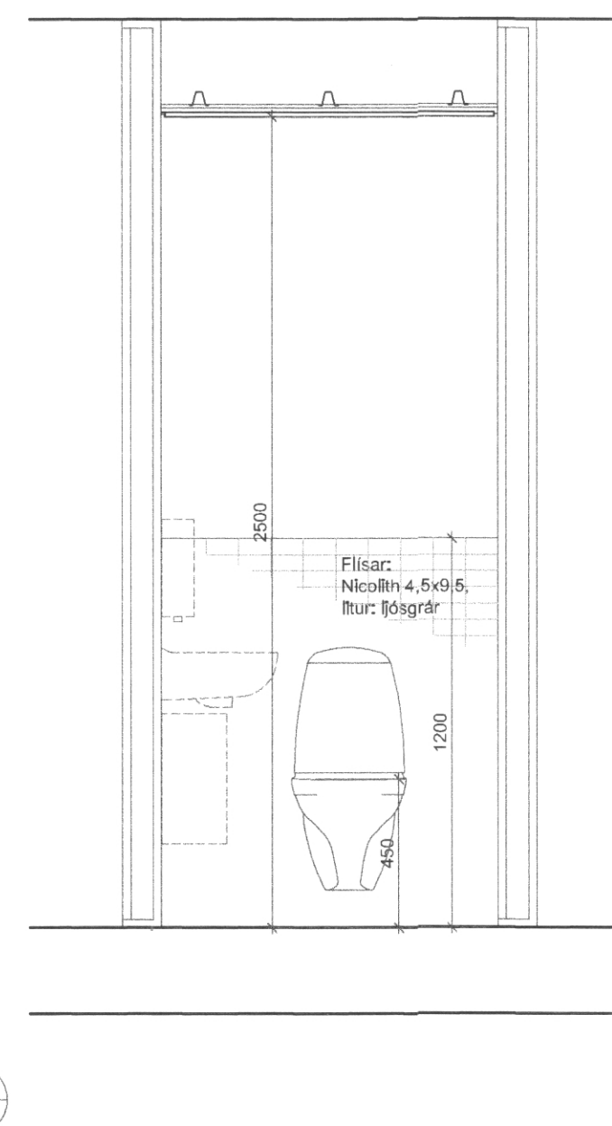
E 70/01 Sneiðing A - A, salerni 1:20
