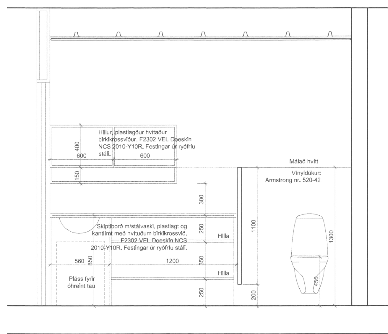
B 70/01 Sneiðing A - A, salerni 1:20
