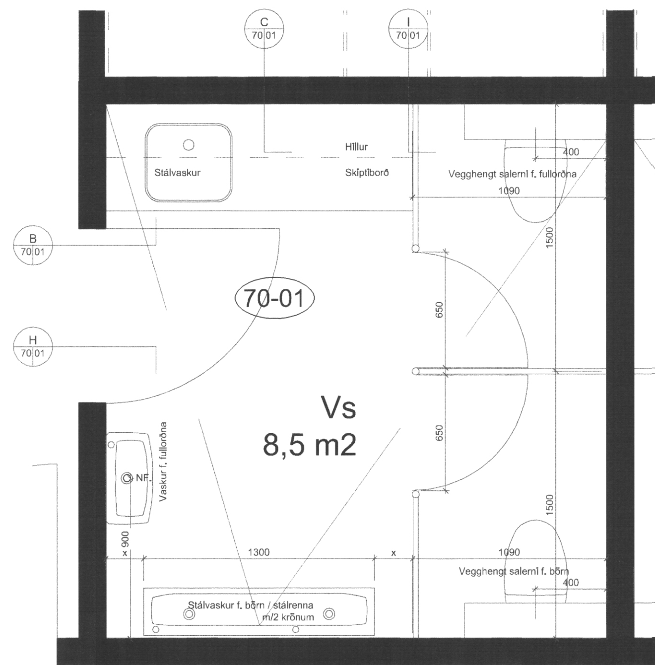
A 70/01 Grunnmynd, salerni Miðheimar 1:20
