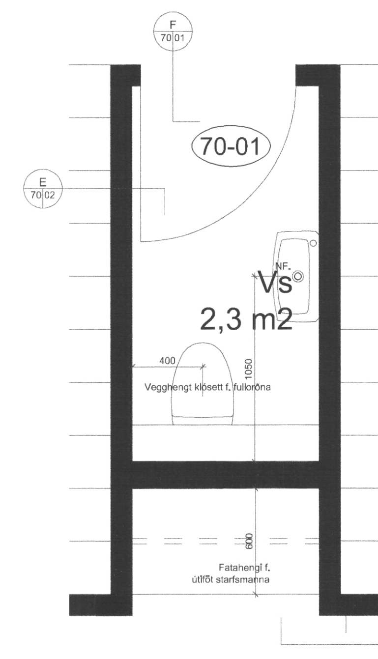
D 70/01 Grunnmynd, salerni 1:20
