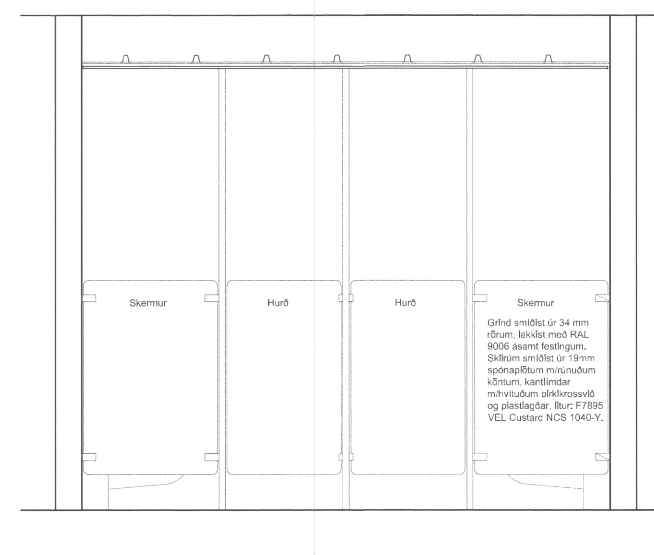
I 70/01 Sneiðing B - B, salerni 1:20
