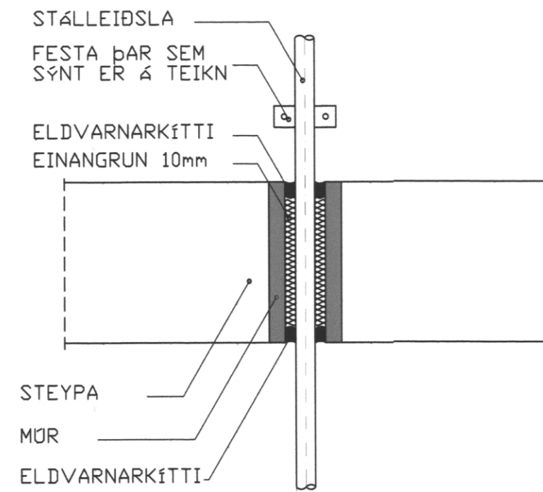
FRÁGANGUR Á STÁLLEIÐSLU GEGNUM STEYPT GÓLF
