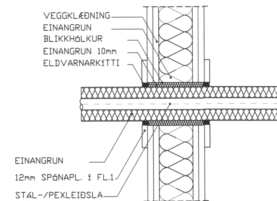
FRÁGANGUR Á STÁL-/PEXLEIÐSLU GEGNUM LÉTTAN VEGG
