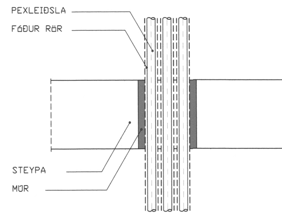
FRÁGANGUR Á PEXLEIÐSLU GEGNUM STEYPT GÓLF
