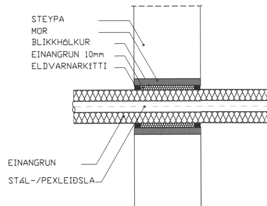
FRÁGANGUR Á STÁL-/PEXLEIÐSLU GEGNUM STEYPTAN VEGG
