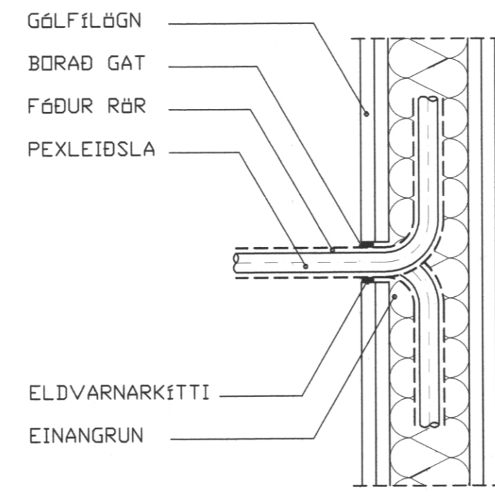
BRUNARÞÉTTING Á PEXLEIÐSLU Í FÁÐURRÖRI Í GEGNUM KLÆÐNINGU
