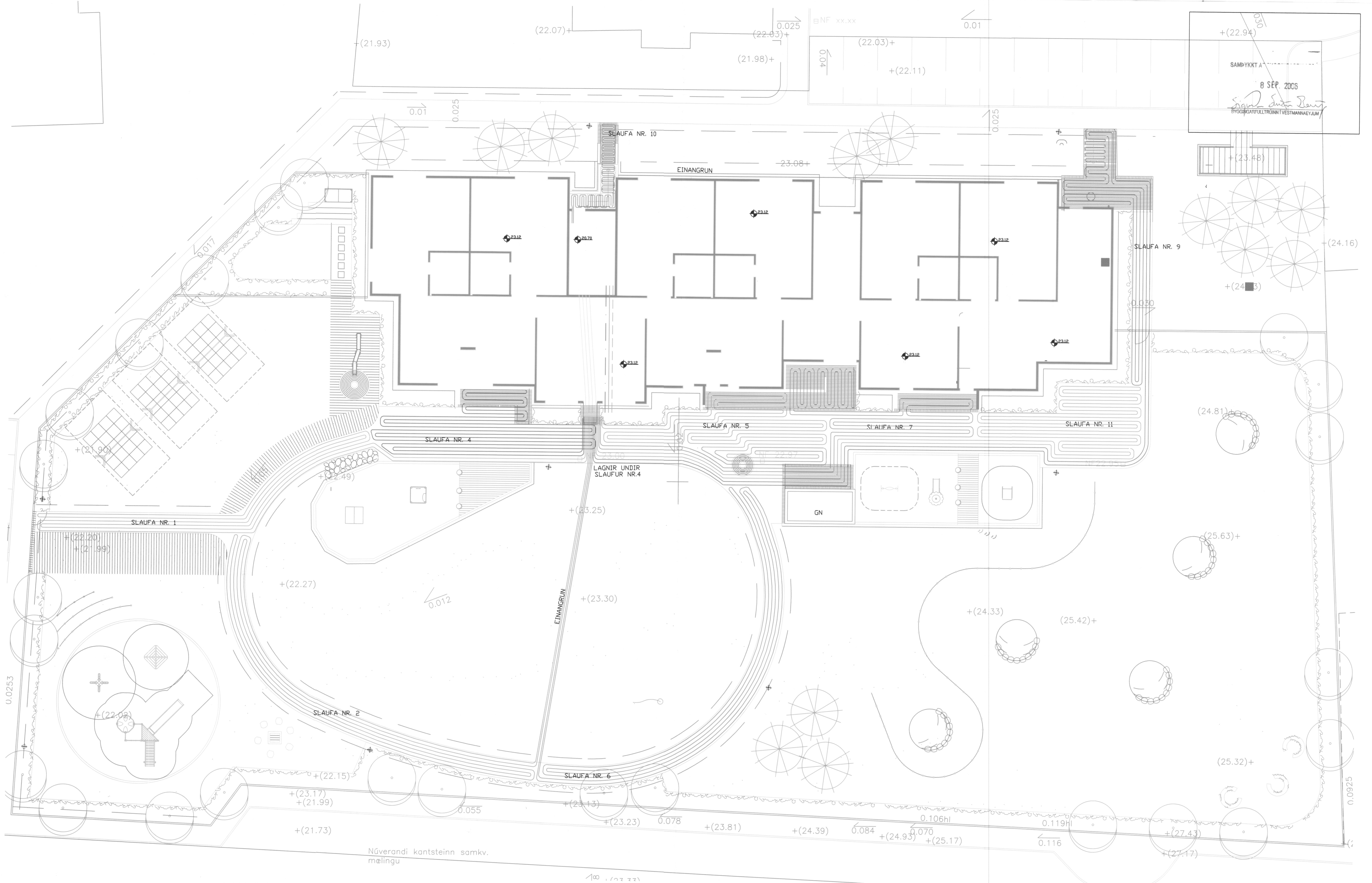
AFSTÖÐUMYND SNJÓBRÆÐSLA M=1:125
