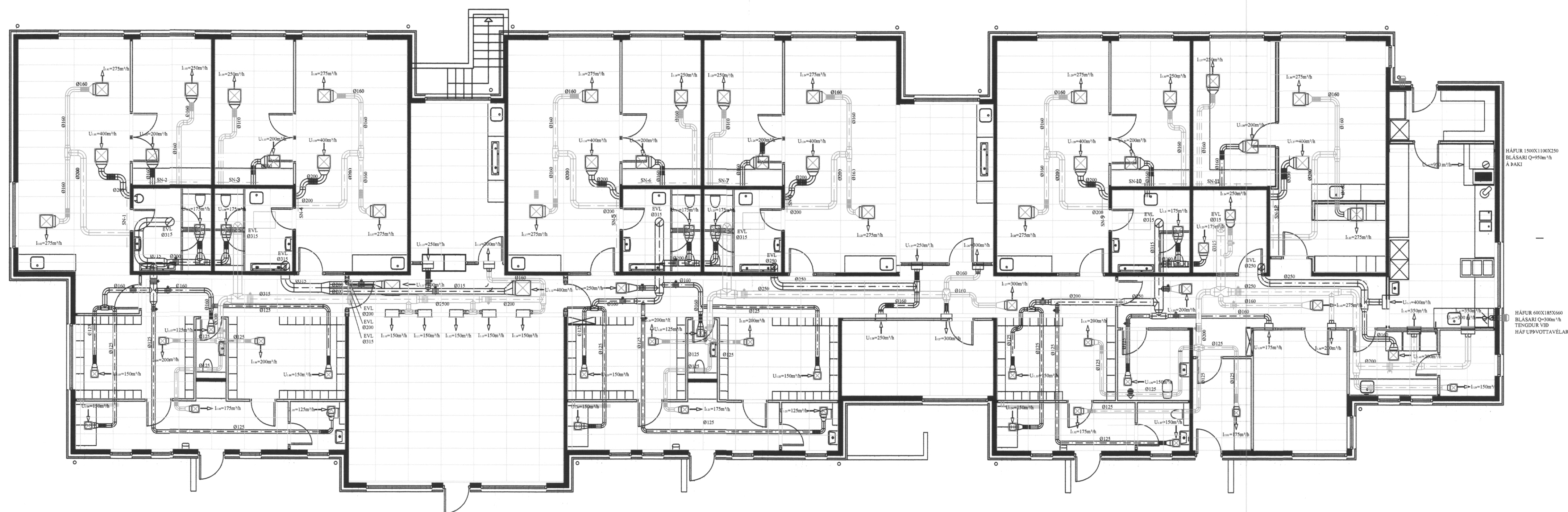
GRUNNMYND 1. HÆÐ LÖFTRÆSING M=1:100
