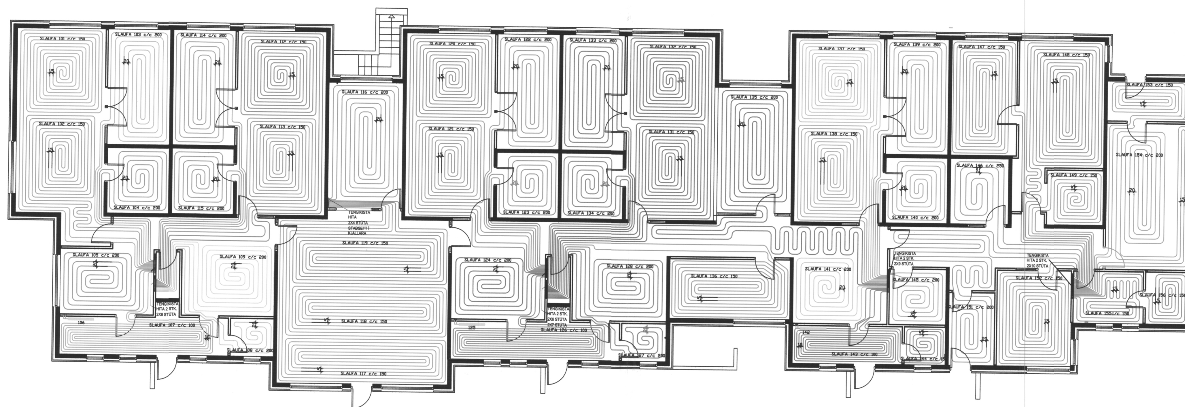
GRUNNMYND 1. HÆÐ HITALAGNA Í PLÖTU M=1:100
