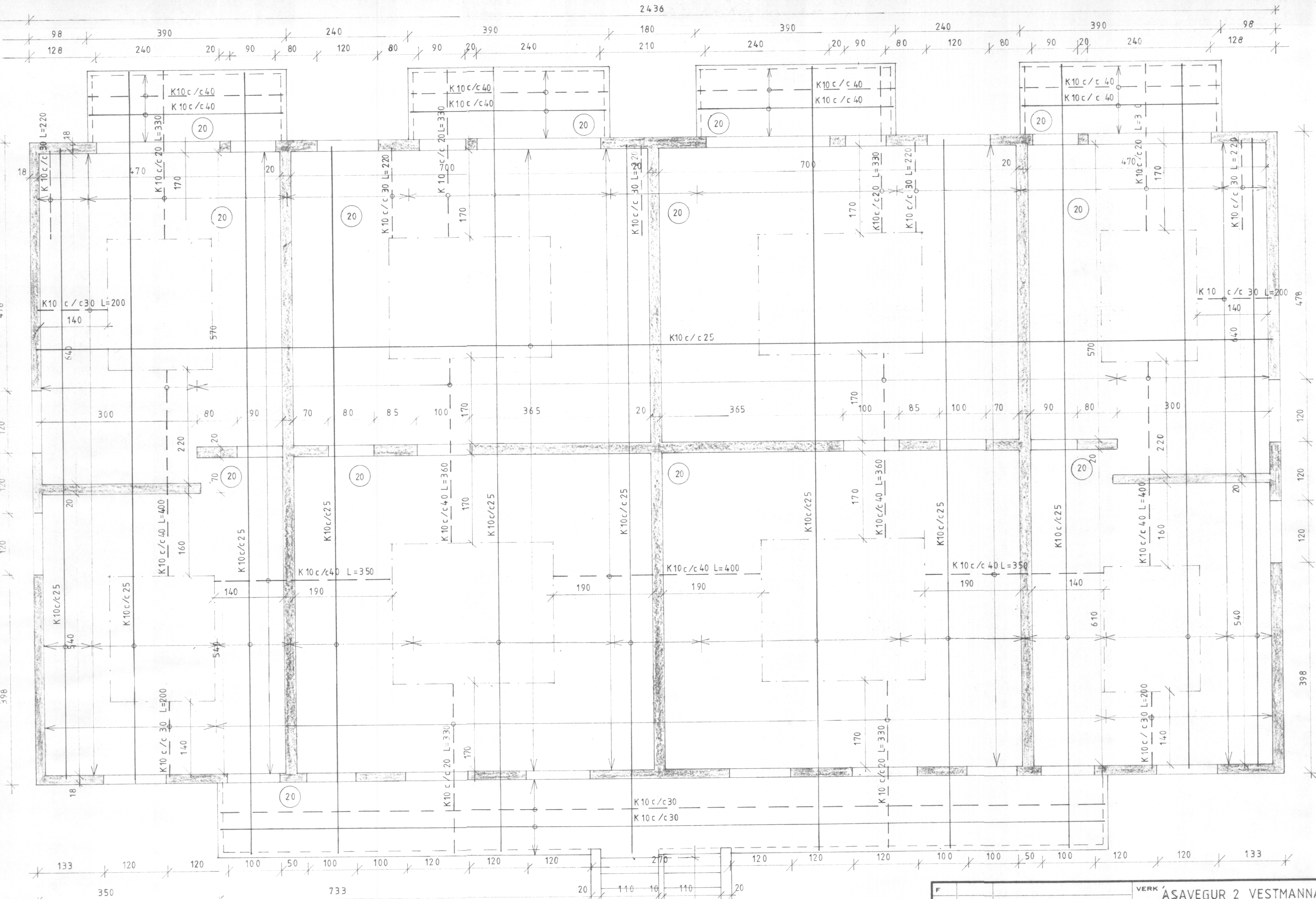
GRUNNMYND 1:50
