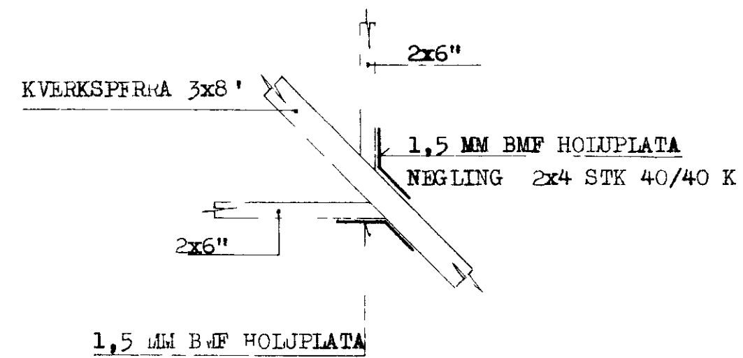
SÉRMYND I 1:20
