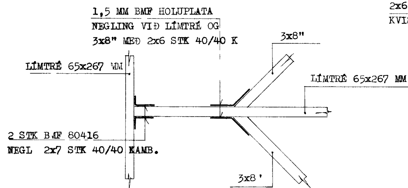
SÉRMYND G 1:20
