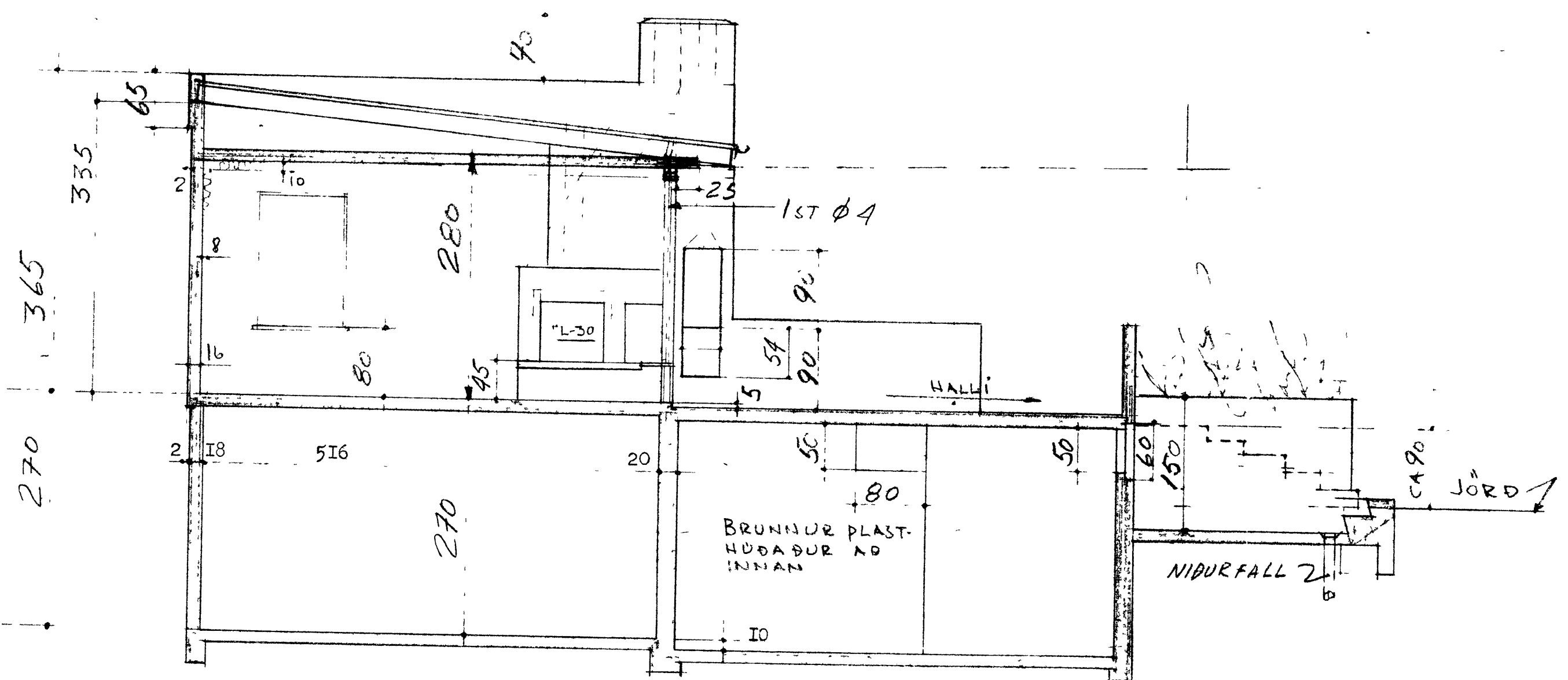
SKURÐUR "A-A"
