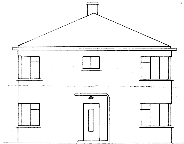
VESTUR
