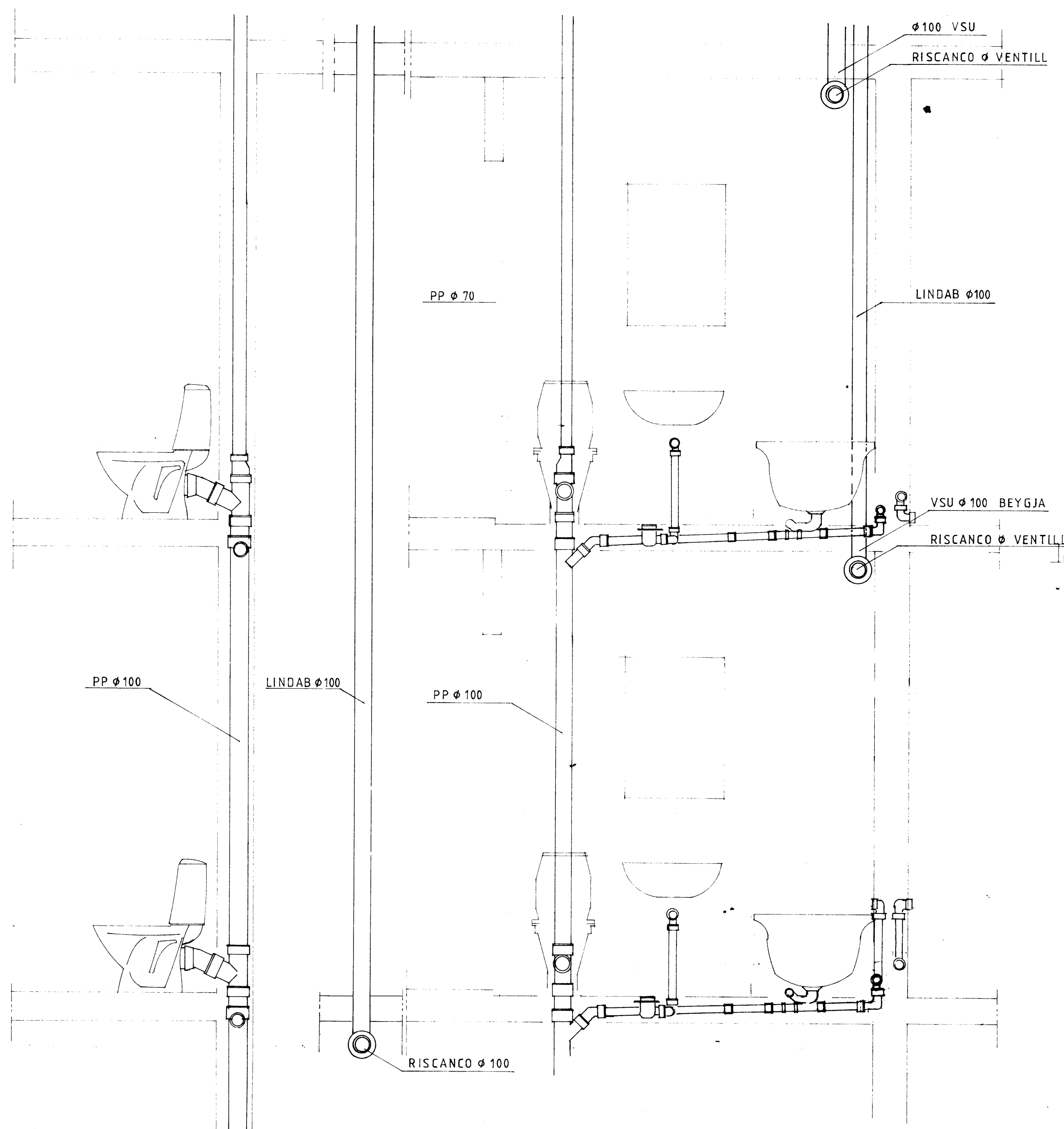
SNID B LOFTRÆSTING FRÁ WC Í KJALLARA SNID A
