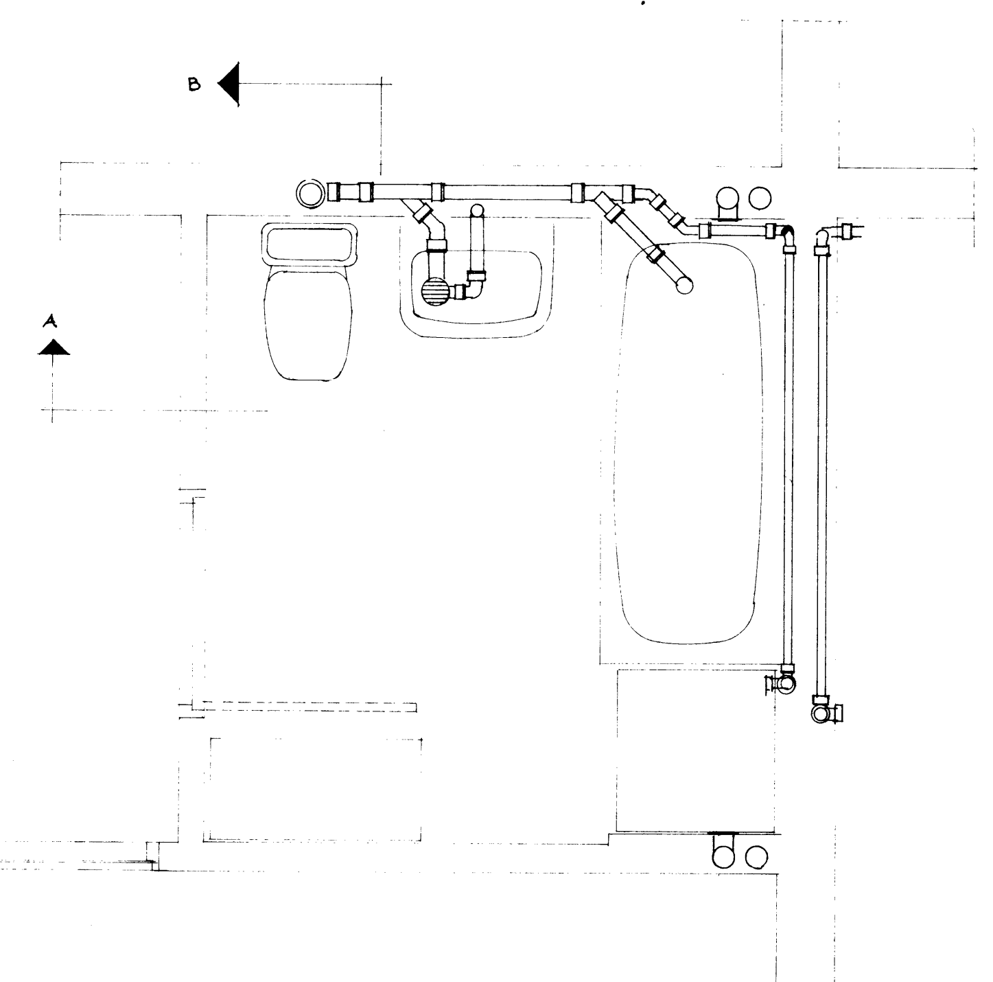
GRUNNMYND 1:20 2 HÆÐ
