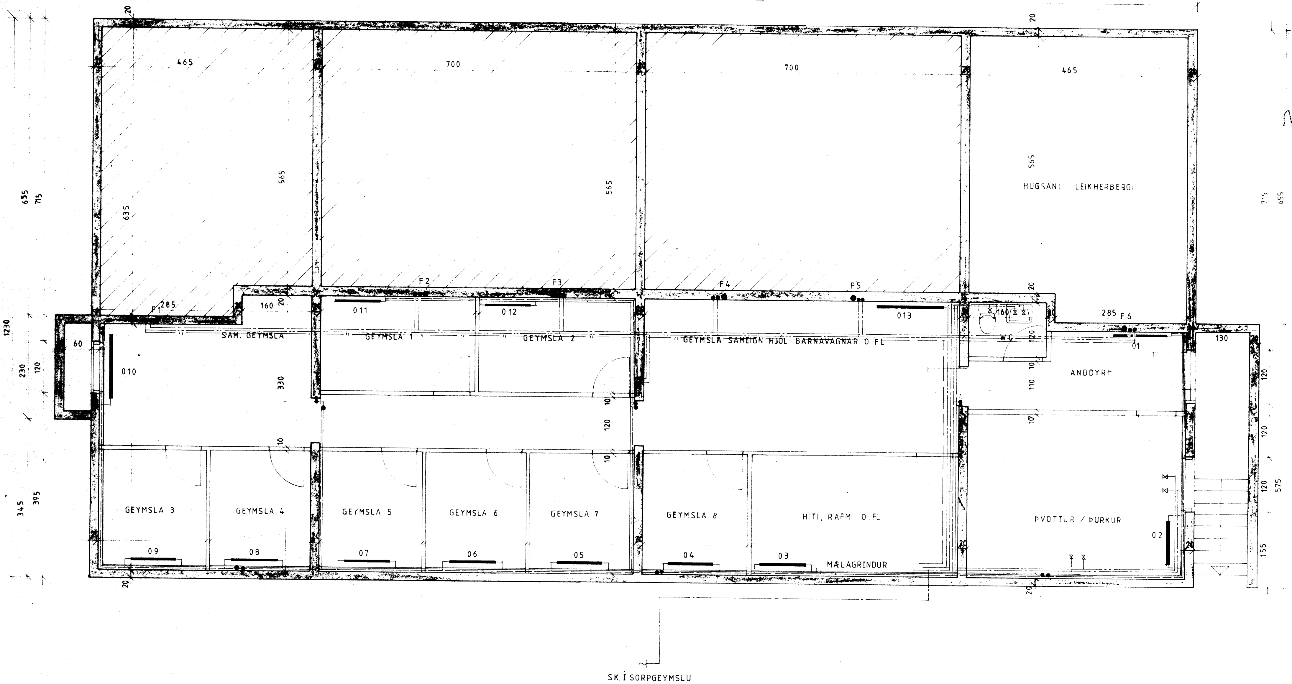
GRUNNMYND KJALLARI 1:50
