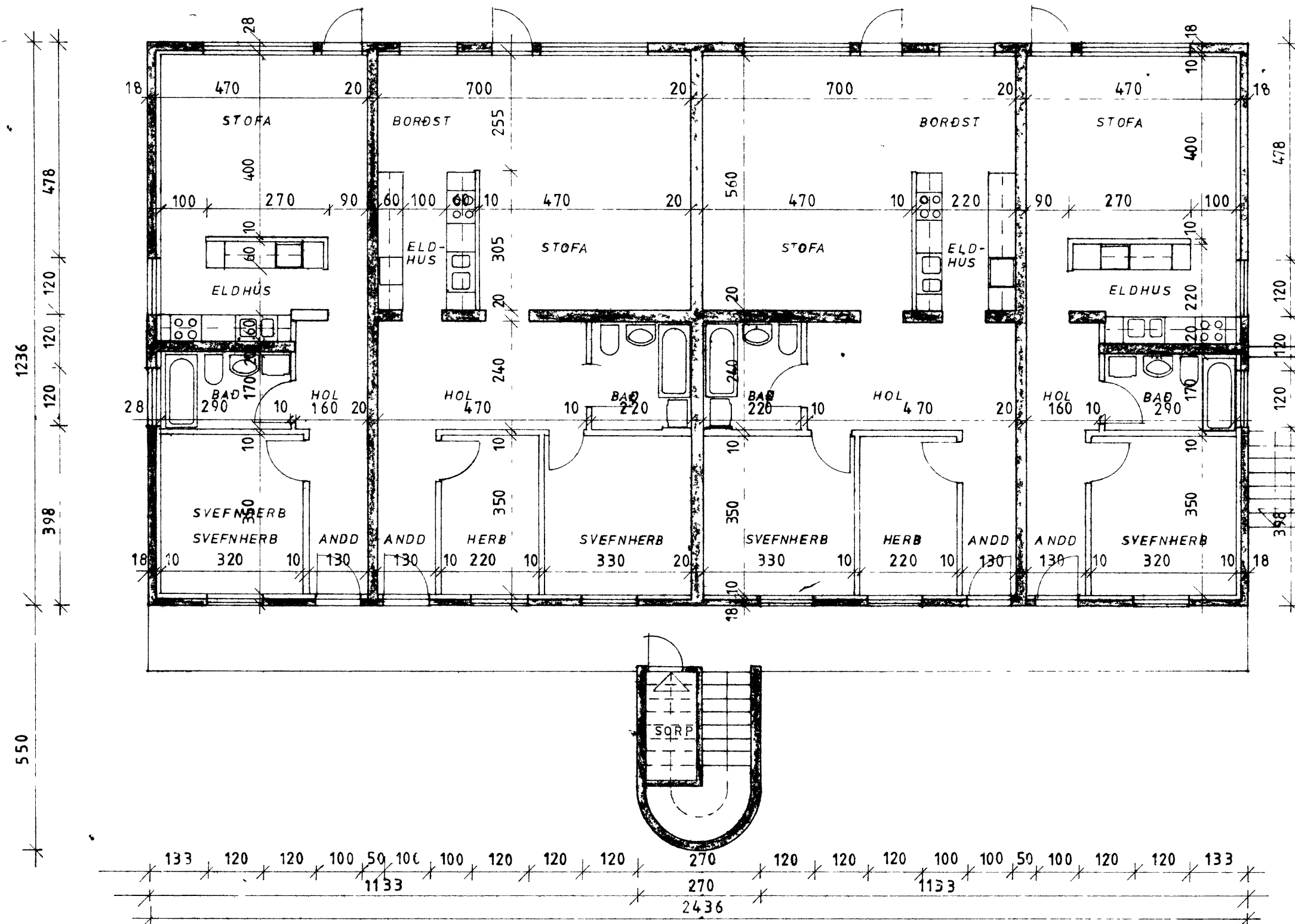
GRUNNMYND 1 HÆÐ 1 100
