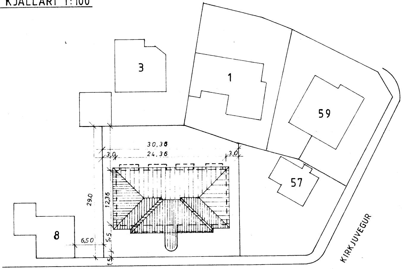
GRUNNMYND KJALLARI 1:100
