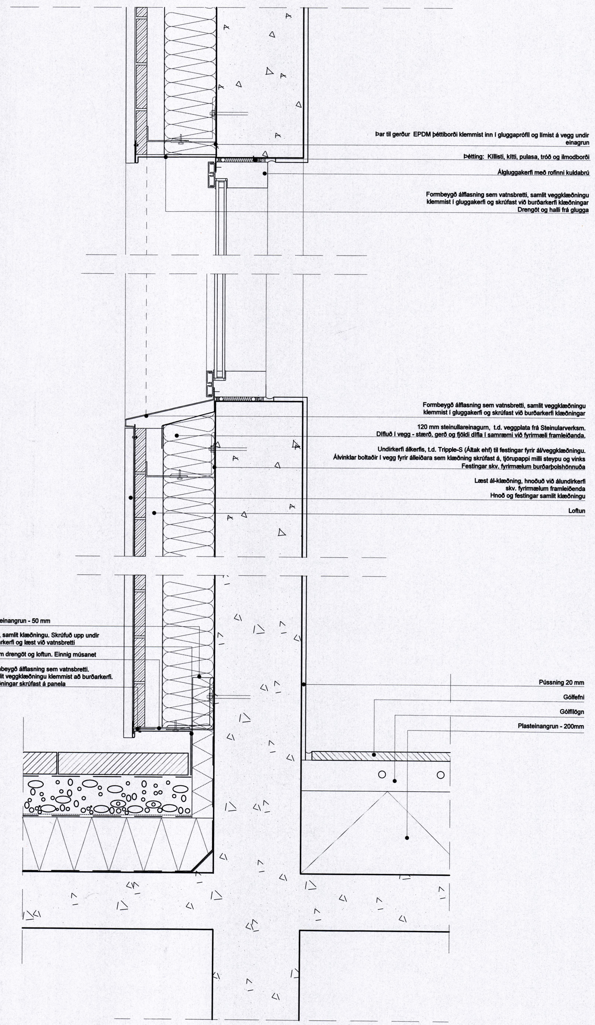
Y1 Lóðrétt deili 210 Útveggur - Gluggi - Sökkull
