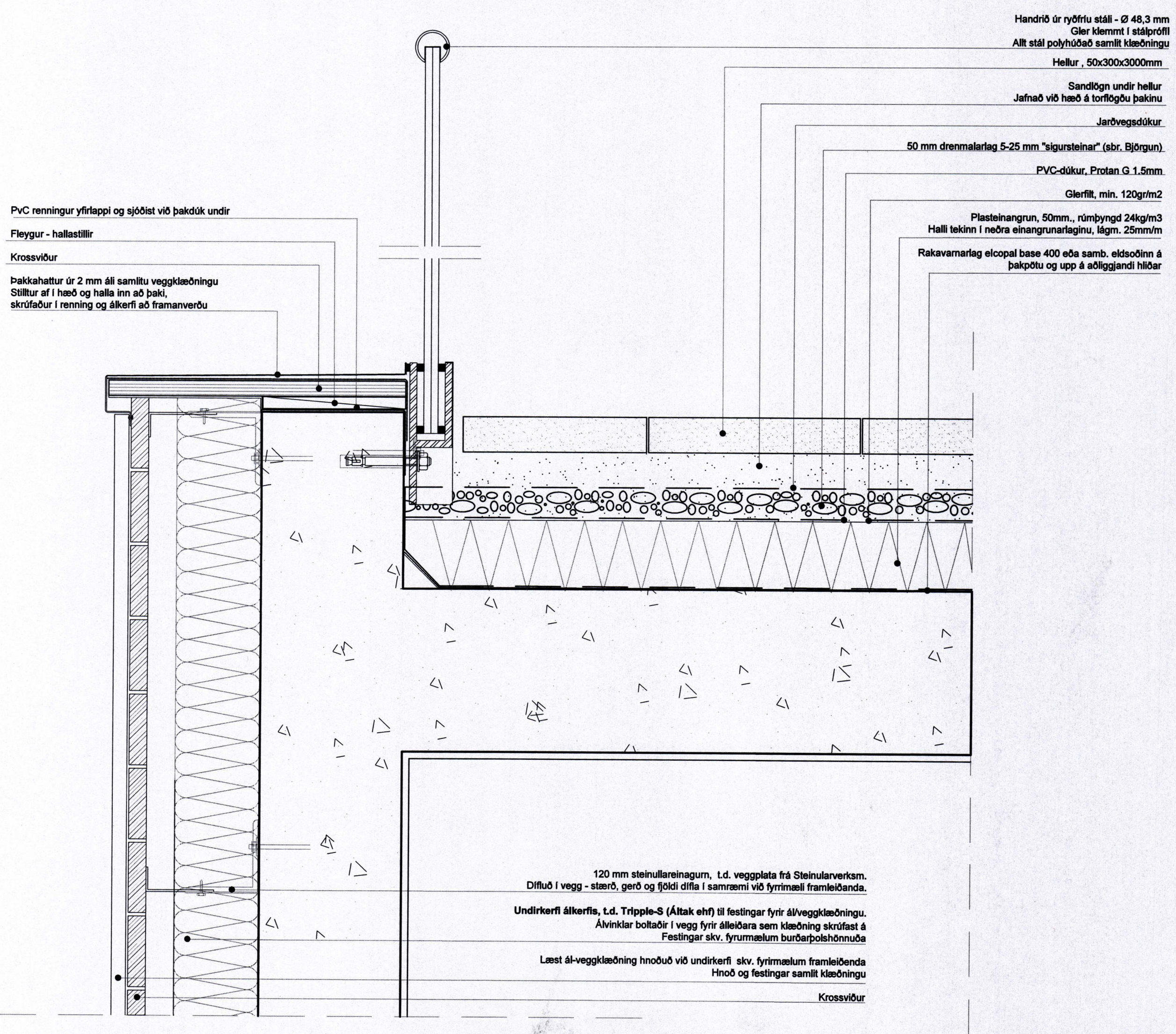
Y2 Lóðrétt deili 210 Garðsvalir
