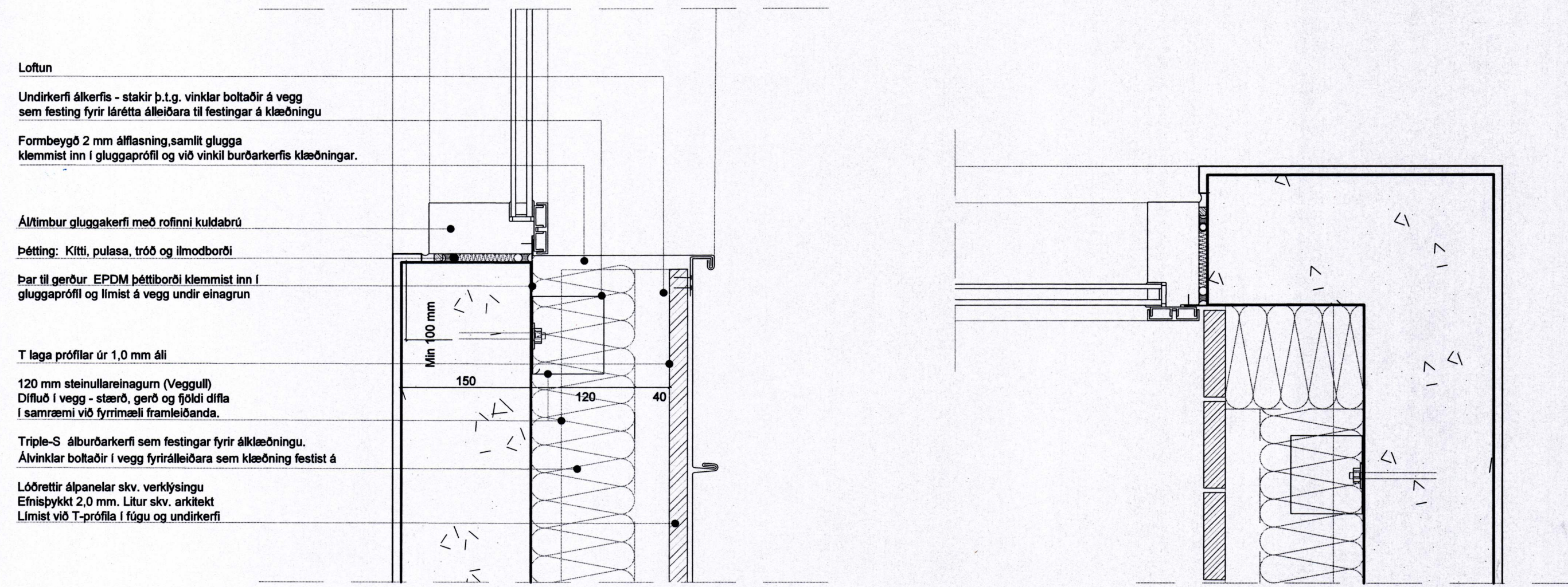
X1 Lárétt deili 201 Útveggur - Gluggi - Álklæðning
